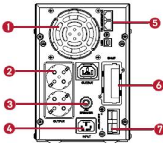
Рисунок 2-2. Вид задней панели ИБП
