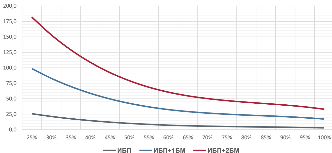
Зависимость времени автономной работы от загрузки ИБП QPS-OLS-RT-2000-49HR
