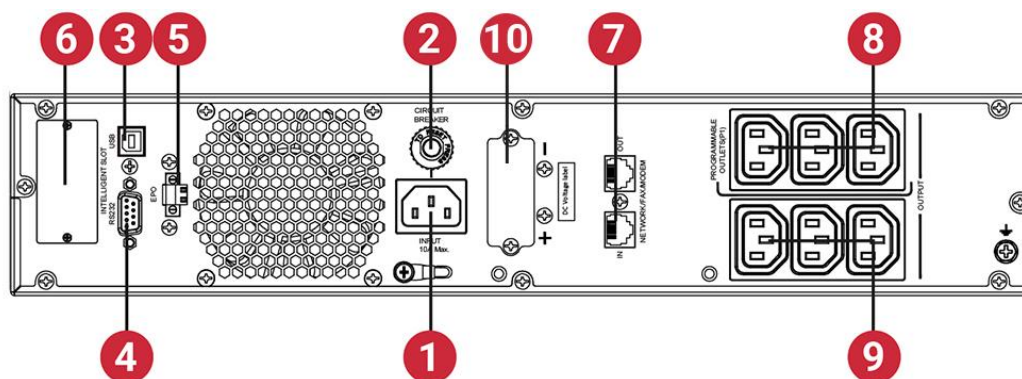
Рисунок 2-1. QPS-OLS-RT-1000-29HR
