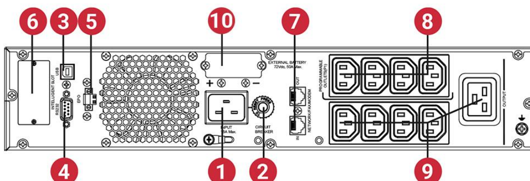
Рисунок 2-3. QPS-OLS-RT-3000-69HR
