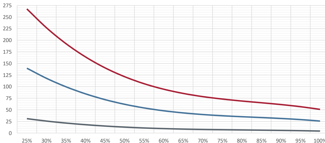
Зависимость времени автономной работы от загрузки ИБП QPS-OLS-RT-1000-29HR
