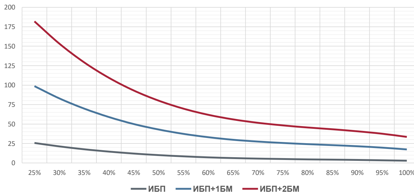
Зависимость времени автономной работы от загрузки ИБП QPS-OLS-RT-3000-69HR
