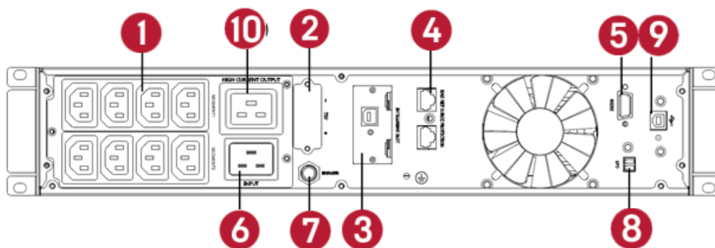
Рисунок 2-3. Вид задней панели ИБП 3 кВ·А
