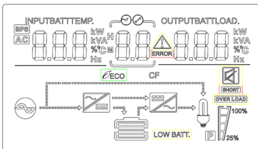
Рисунок 2-18. Индикаторы на ЖК-дисплее
