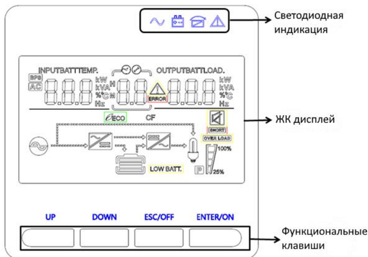
Рисунок 2-17. Внешний вид панели управления
