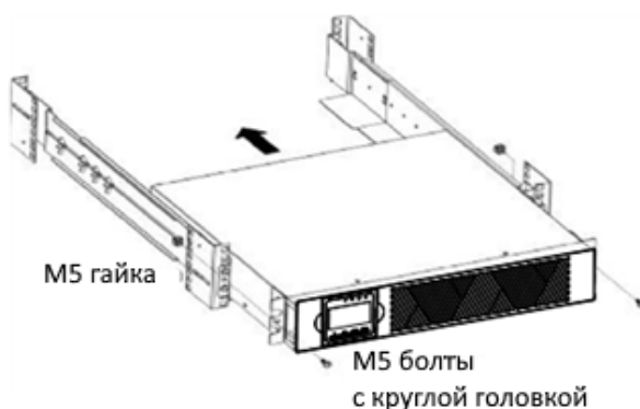
Рисунок 2-7. Установка и крепление ИБП в стойке
