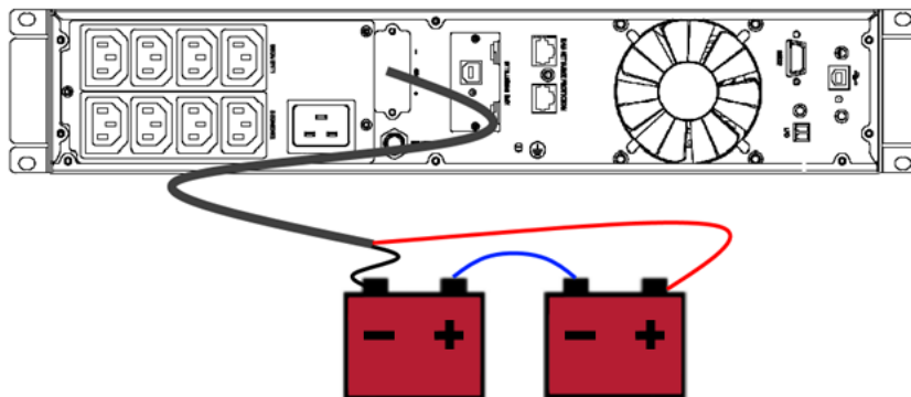
Рисунок 2-13. Подключение внешних аккумуляторных батарей
