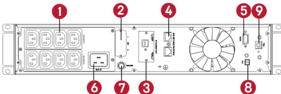
Рисунок 2-1. Вид задней панели ИБП 1 кВ·А и 1,5 кВ·А
