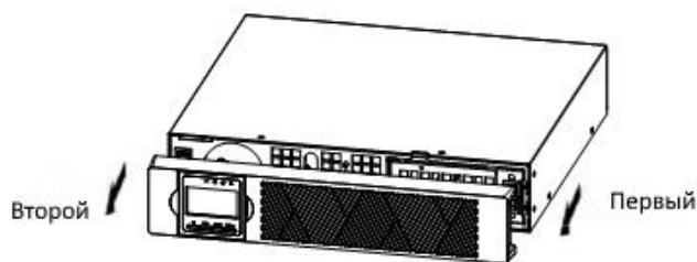
Рисунок 2-8. Снятие передней крышки ИБП
