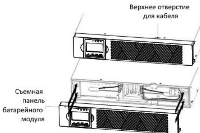
Рисунок 2-10. Установка передней крышки ИБП
