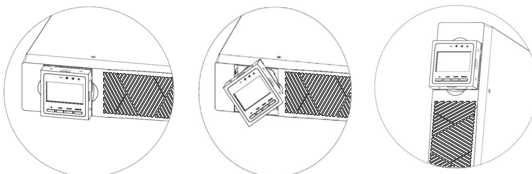
Рисунок 2-16. Установка дисплея для вертикального использования
