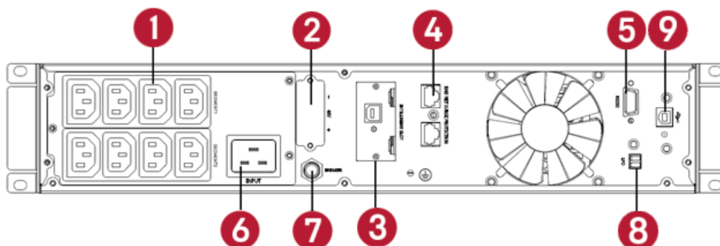
Рисунок 2-2. Вид задней панели ИБП 2 кВ·А
