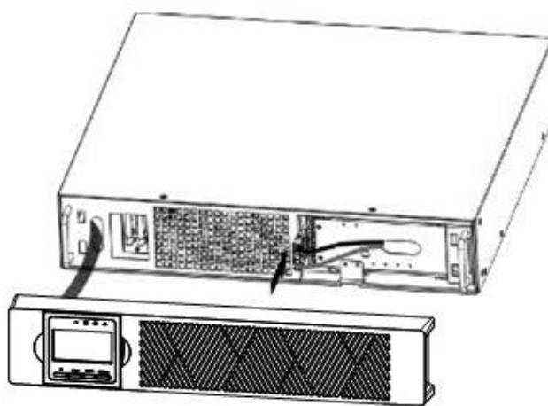
Рисунок 2-9. Подключение внутренних батарей
