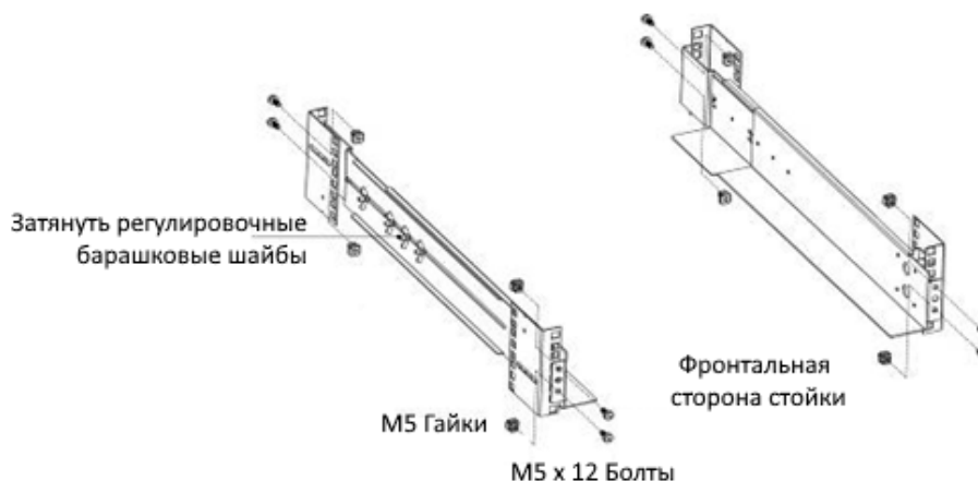
Рисунок 2-5. Крепление монтажного комплекта рельс
