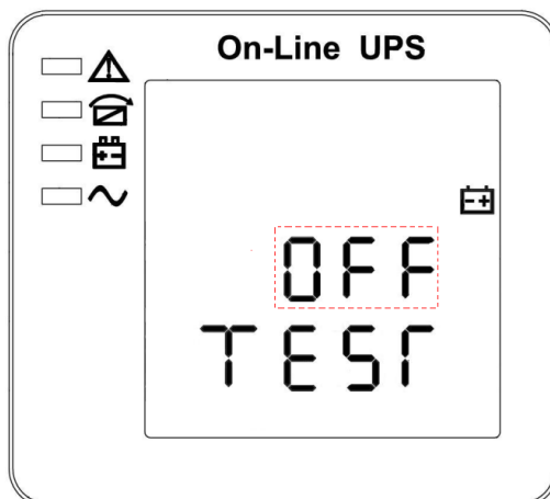
Рисунок 18. Настройка тестирования АКБ (Примечание: изображение, выделенное пунктиром, мигает)
