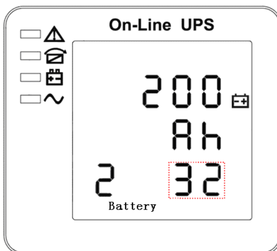
Рисунок 14. Настройка количества АКБ (Примечание: изображение, выделенное пунктиром, мигает)
