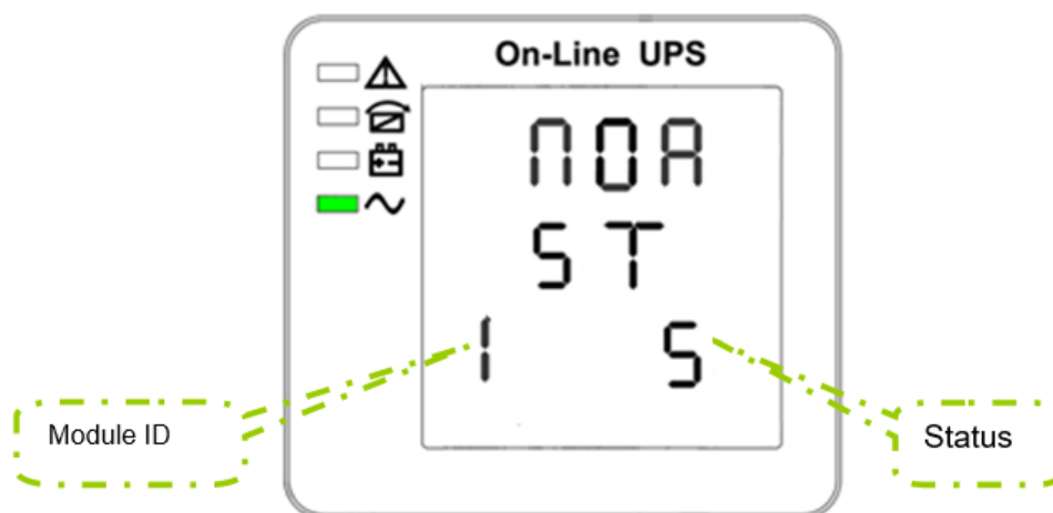
Рисунок 9. Интерфейс рабочего состояния и режима работы ИБП
