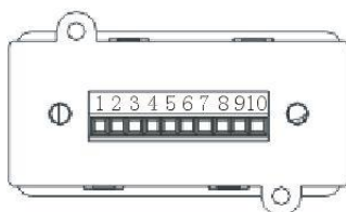
Рисунок 24. Внешний вид платы сухих контактов
