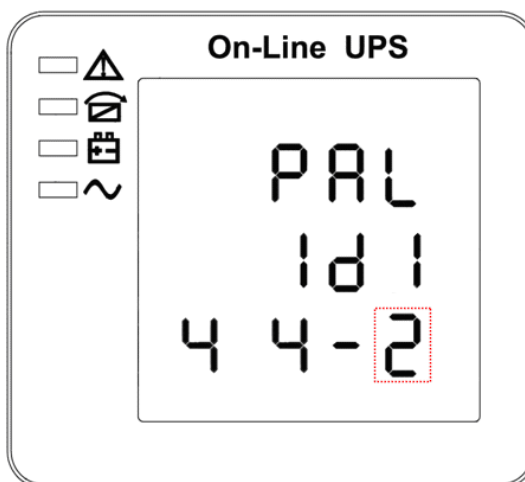
Рисунок 23. Меню настройки количества резервных модулей (Примечание: изображение, выделенное пунктиром, мигает)
