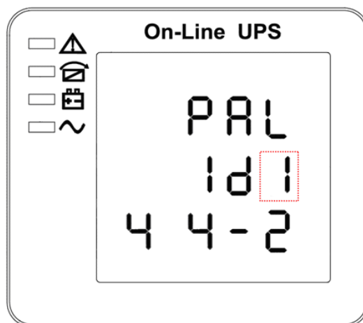
Рисунок 21. Меню настройки идентификатора при параллельной работе ИБП (Примечание: изображение, выделенное пунктиром, мигает)
