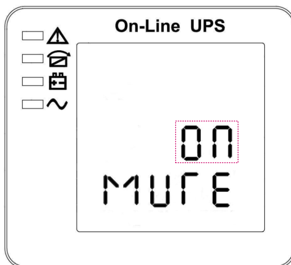
Рисунок 17. Настройка отключения звука (Примечание: изображение, выделенное пунктиром, мигает)
