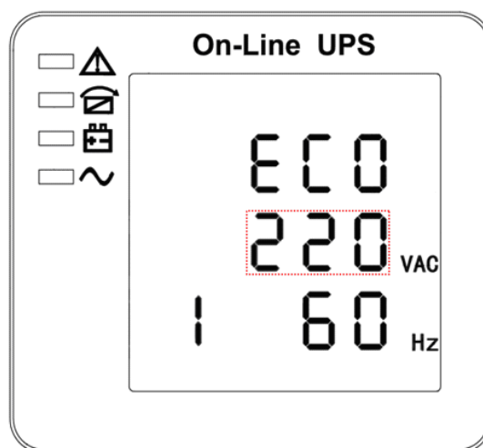
Рисунок 11. Настройка выходного напряжения (Примечание: изображение, выделенное пунктиром, мигает)
