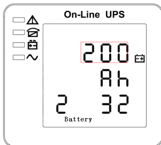
Рисунок 13. Настройка ёмкости батареи (Примечание: изображение, выделенное пунктиром, мигает)
