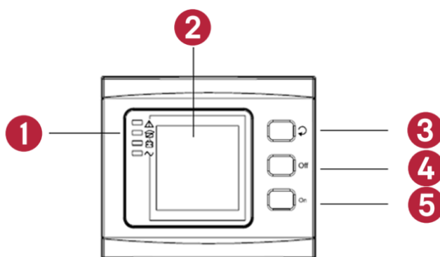
Рисунок 4. Панель управления и ЖК-дисплей
