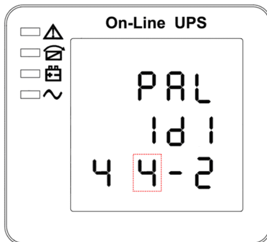
Рисунок 22. Меню настройки количества параллельных модулей (Примечание: изображение, выделенное пунктиром, мигает)
