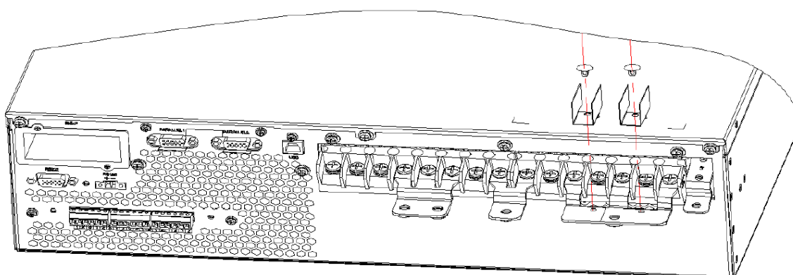
Рисунок 3-18. Установка изоляционной пленки
