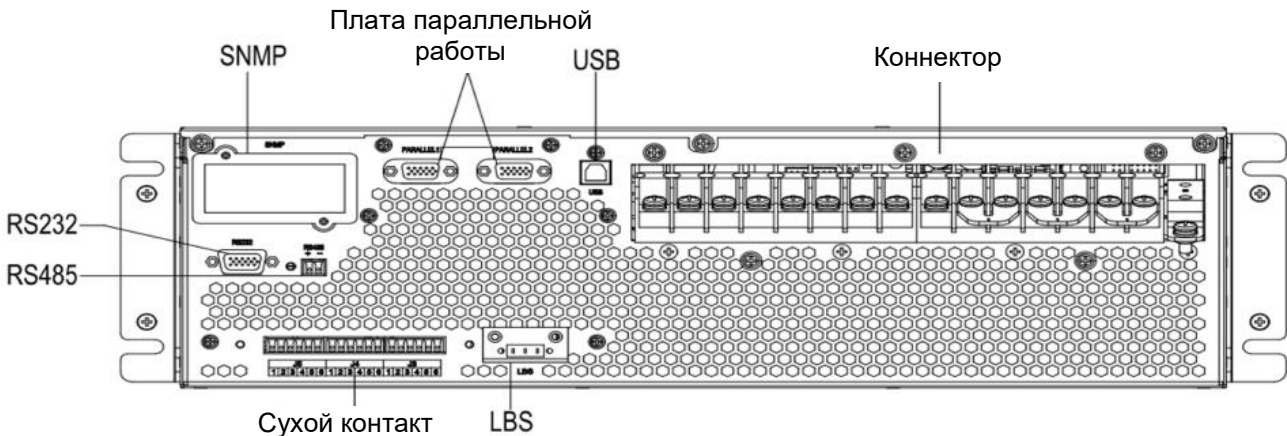
Рисунок 3-21. Сухие контакты и коммуникационные интерфейсы
