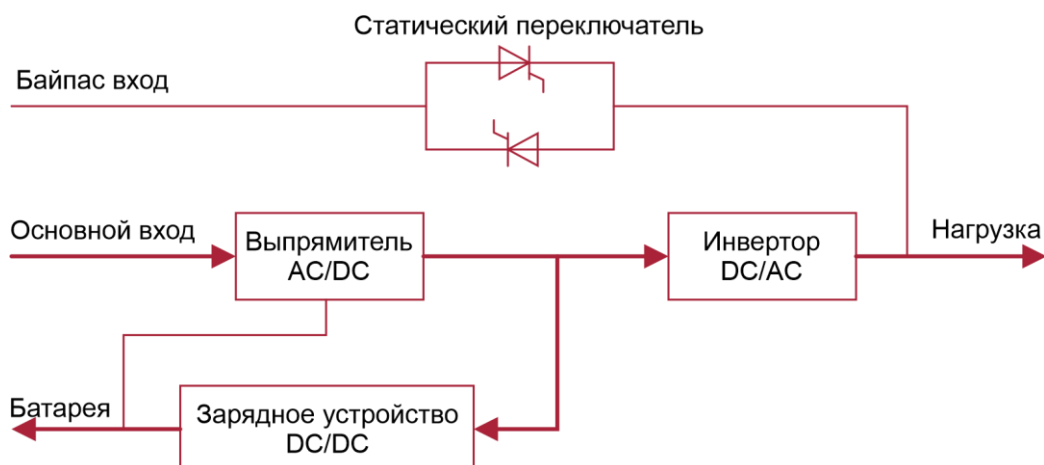
Рисунок 3-32. Нормальный режим
