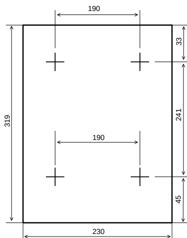
Рисунок 2. Габаритно-установочные размеры
