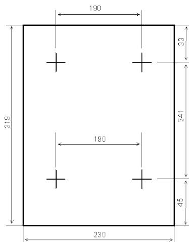
Рис. 2. Габаритно-установочные размеры
