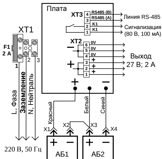
Рис. 3. Схема подключения
