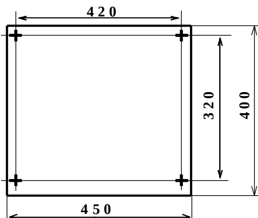
Рисунок 1. Габаритно-установочные размеры
