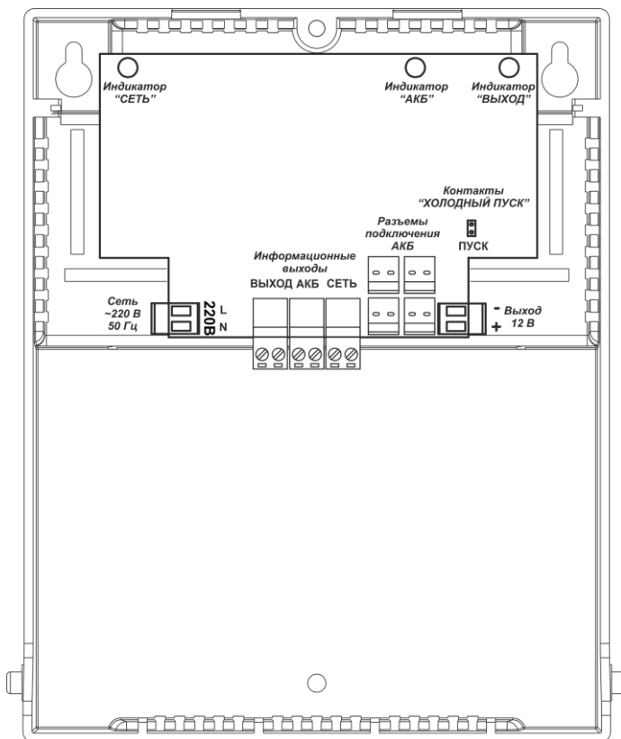
Рисунок 1 – Вид изделия со снятой крышкой
