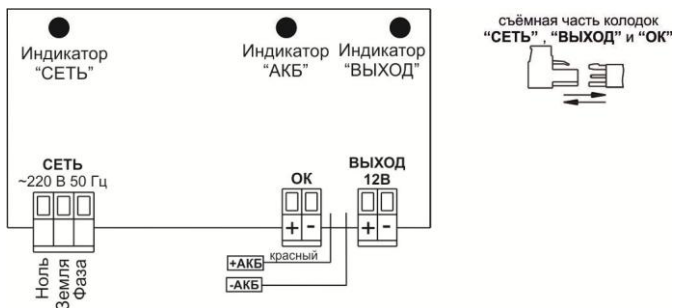
Рисунок 1 - Вид изделия с открытой крышкой (схема подключения)
