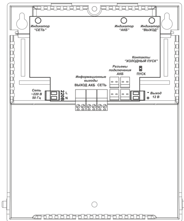
Рисунок 1 – Вид изделия со снятой крышкой
