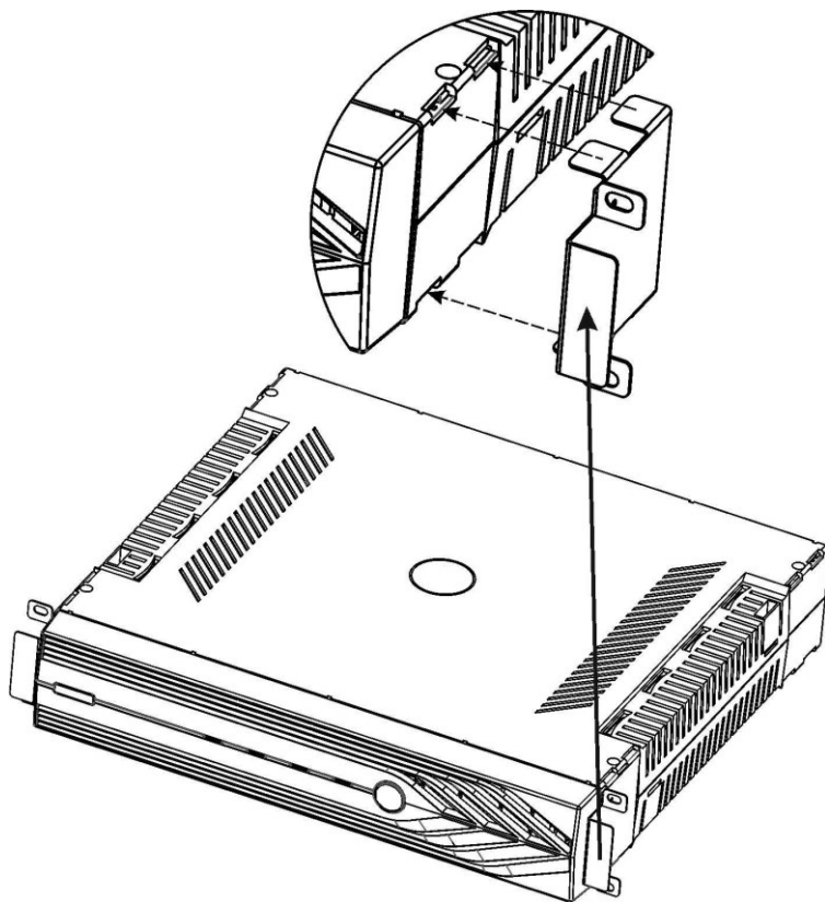
Рисунок 3 – Крепление кронштейнов для установки изделия в 19" стойку
