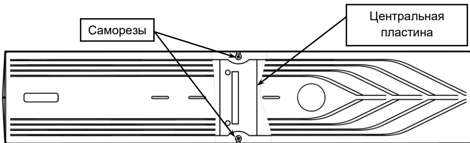
Рисунок 6 – Крепление центральной фиксирующей пластины
