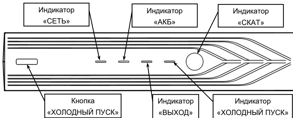
Рисунок 1 — Общий вид передней панели источника
