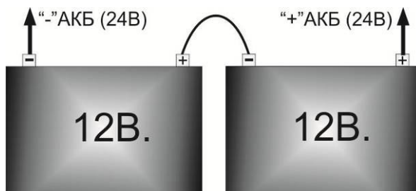
Рисунок 4 – схема последовательного соединения двух аккумуляторов
