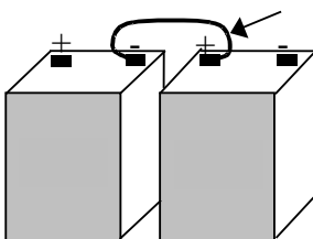
Рисунок 6 – Схема соединения аккумуляторов
