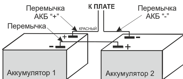
Рисунок 3 – подключение АКБ
