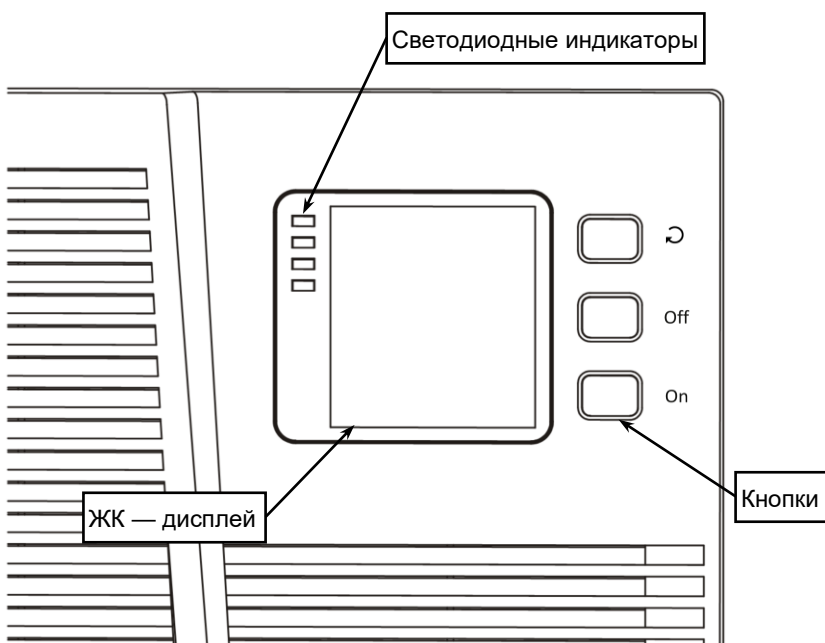
Рисунок 2 — Общий вид передней панели изделия
