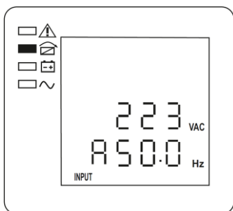
Рисунок 6 — ЖК-дисплей, Фаза А, входное напряжение и частота
