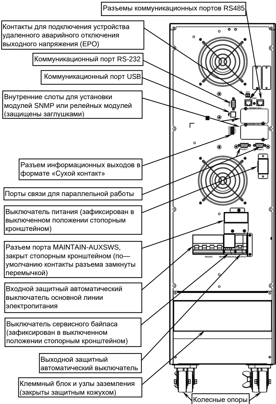
Рисунок 3 — Общий вид задней панели изделия
