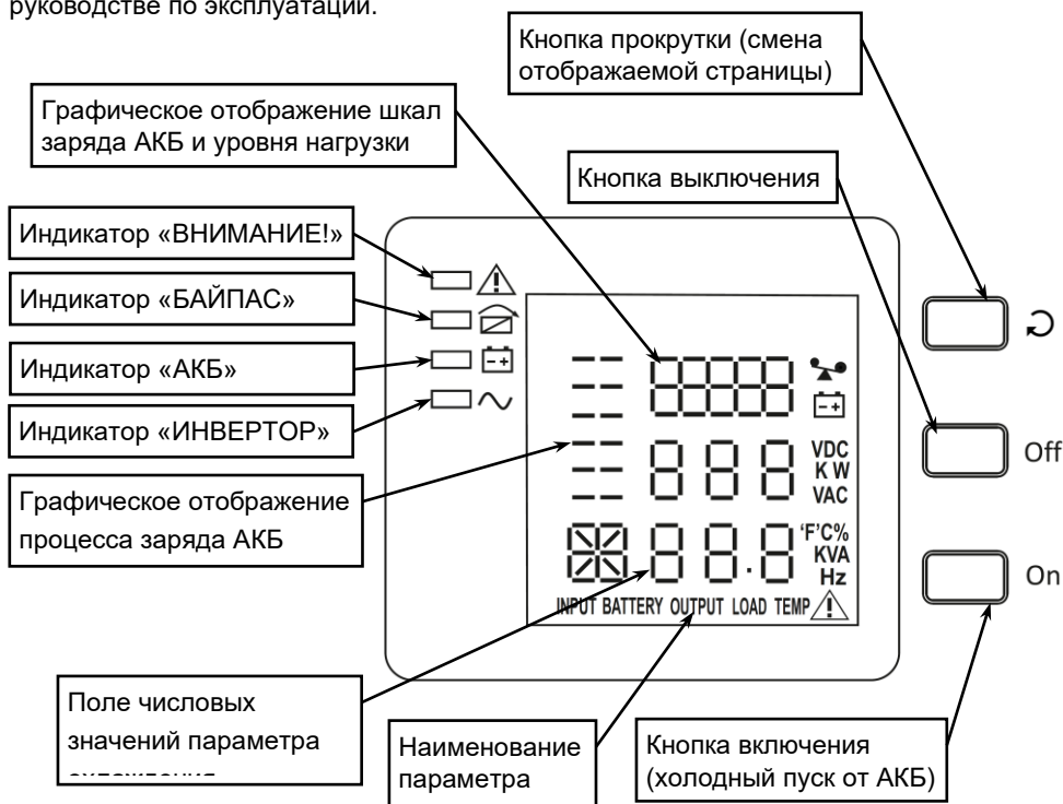
Рисунок 4 — Описание ЖК—дисплея
