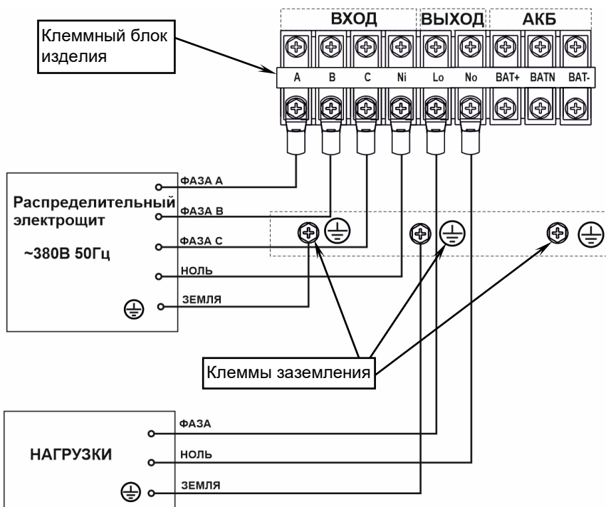
Рисунок 19 — Схема подключения изделия и монтажа аккумуляторной батареи
