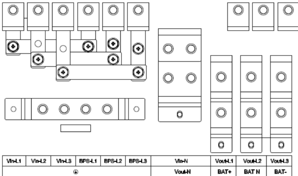
Рисунок 6 – Схема подключения изделия при одиночном входе для SKAT-UPS 100-3/3-ON, где клеммы Vin и BPS соединены медными перемычками по фазам и нейтрали
