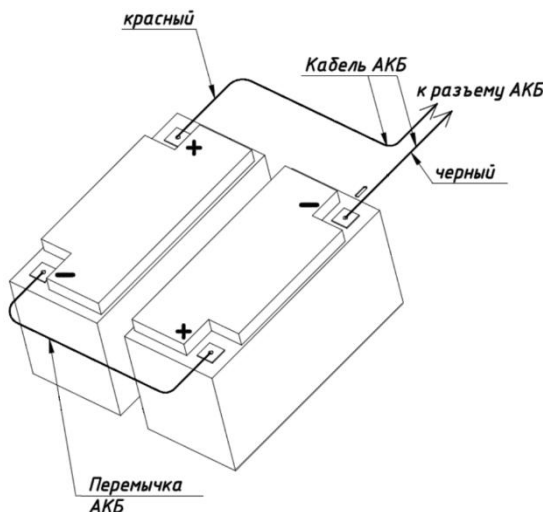
Рисунок 13 — Схема монтажа аккумуляторной батареи
