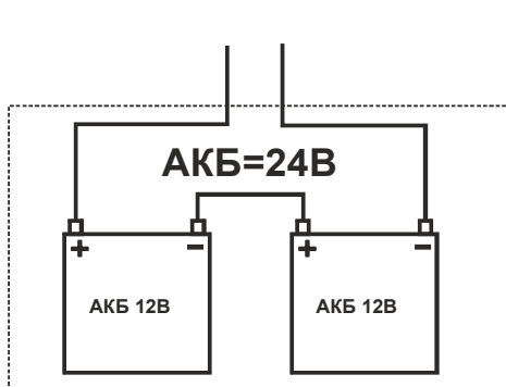
Схема монтажа аккумуляторной батареи для SKAT-UPS 1000-RACK-ON P3 и SKAT-UPS 1000-RACK-ON-E P3
