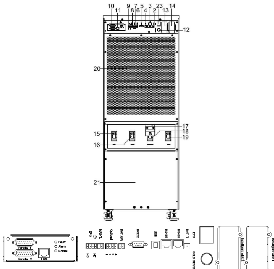
Рисунок 2 – Общий вид задней панели изделия, где
