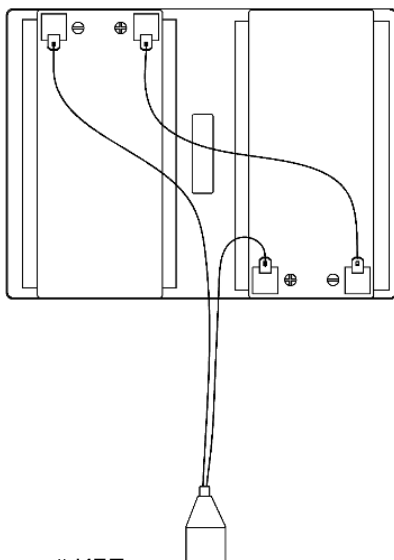
Рисунок 13 Подключение внутренних батарей ИБП SKAT-UPS 1000-RACK-ON-2x9-IS исп.Л
