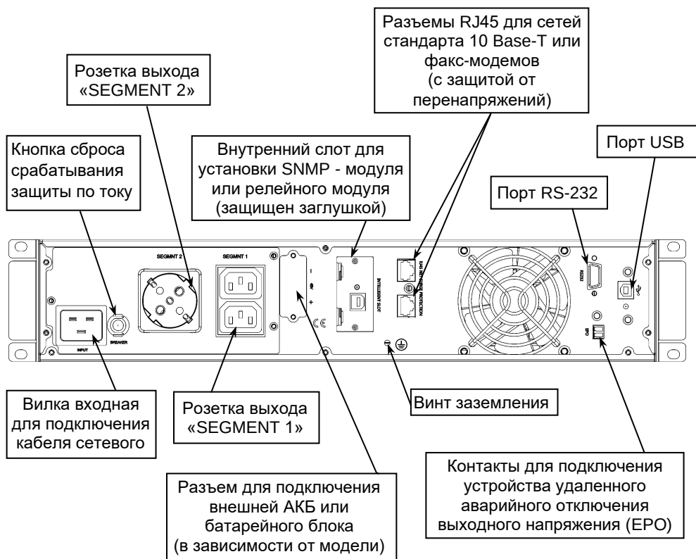
Рисунок 3 – Общий вид задней панели SKAT-UPS 2000-RACK-ON-4x9-IS исп.Л, SKAT-UPS 2000-RACK-ON-IS исп.Л
