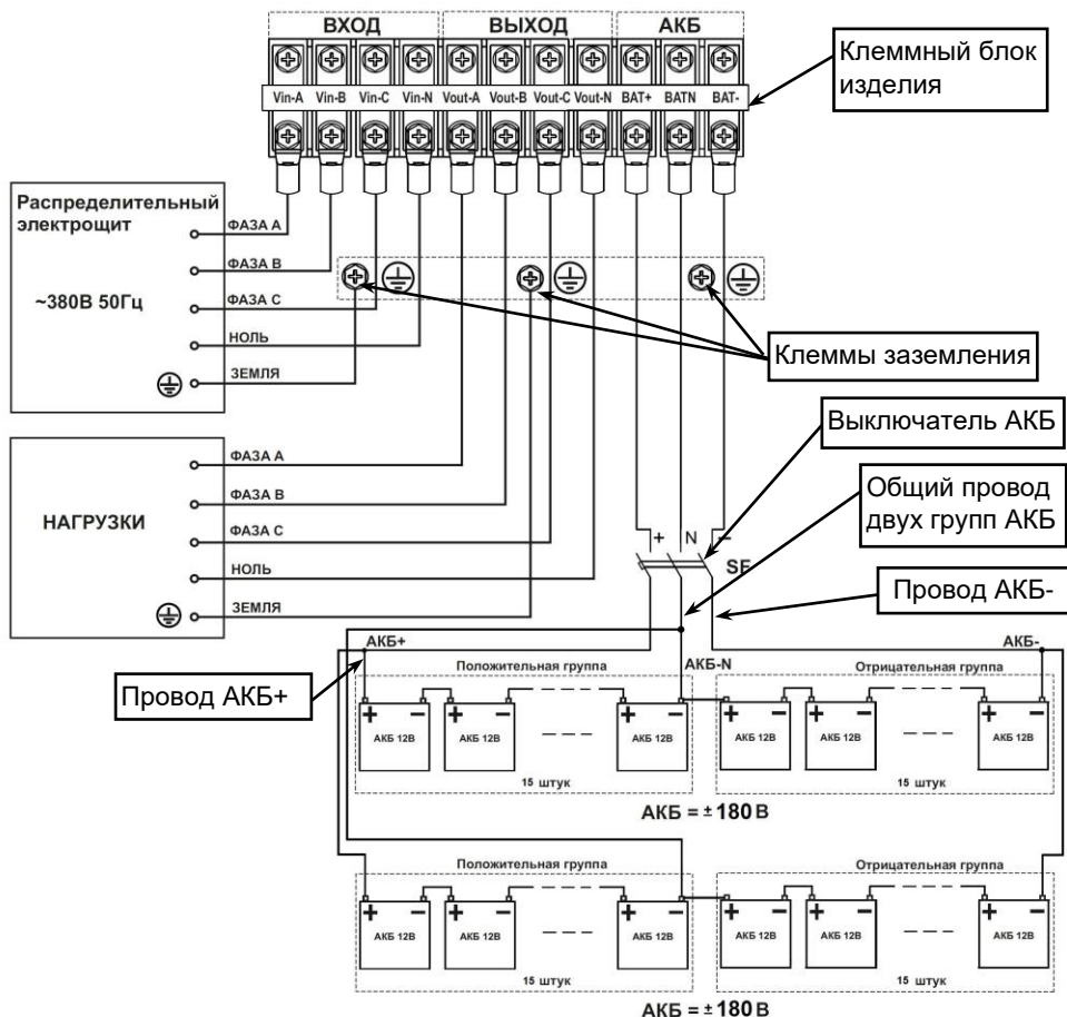
Рисунок 23.4 – Схема подключения изделия и монтажа внешних аккумуляторных батарей для SKAT-UPS 40-3/3-ON-2x(30x9)
