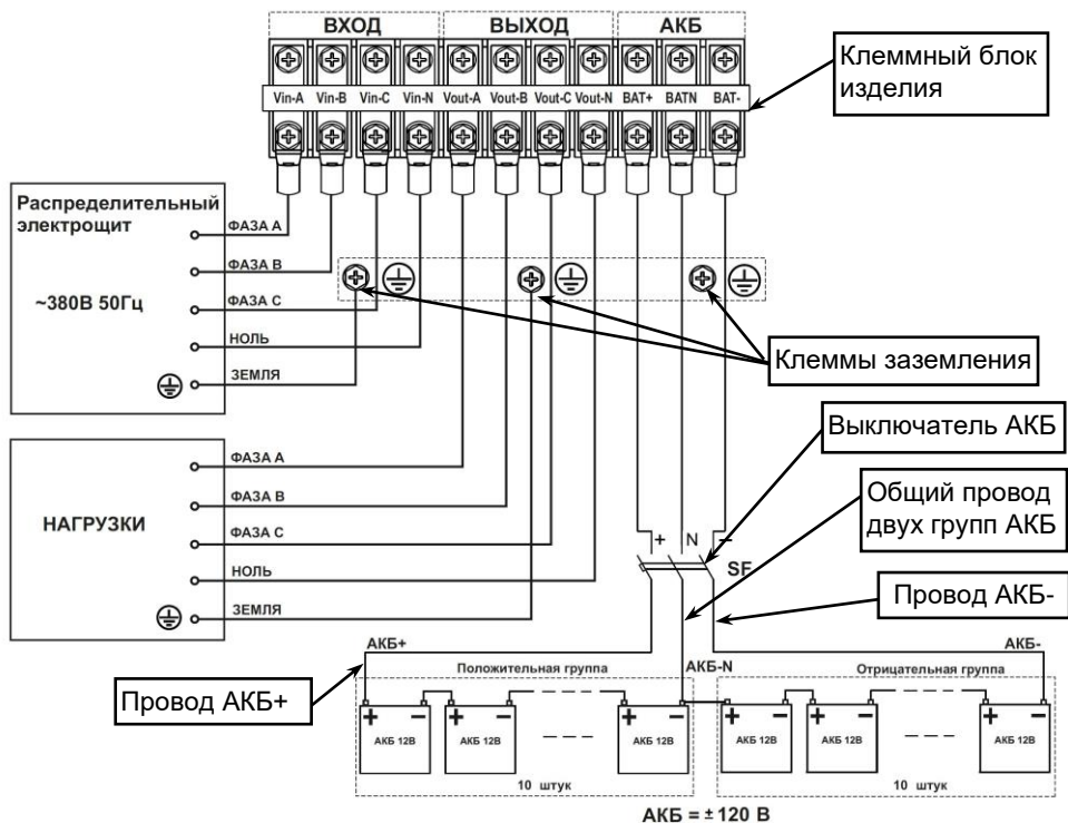
Рисунок 23.1 – Схема подключения изделия и монтажа внешних аккумуляторных батарей для SKAT UPS 10-3/3-ON-20x9
