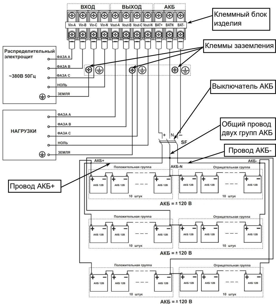
Рисунок 23.3 – Схема подключения изделия и монтажа внешних аккумуляторных батарей для SKAT-UPS 30-3/3-ON-3x(20x9)
