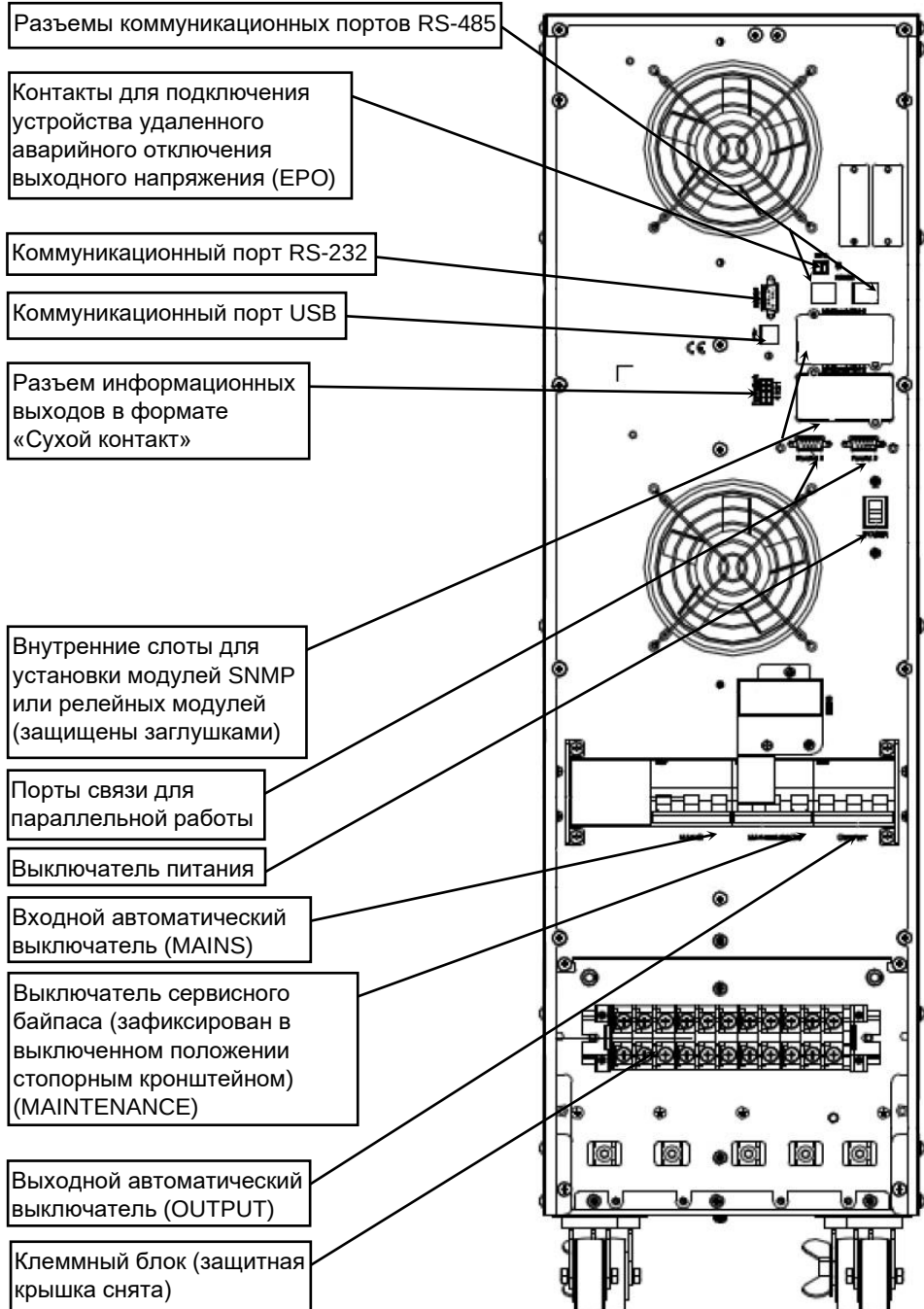
Рисунок 2.1 – Общий вид задней панели изделий SKAT-UPS 10-3/3-ON-(20x9) и SKAT-UPS 10-3/3-ON-2x(20x9) со снятой крышкой клеммного блока
