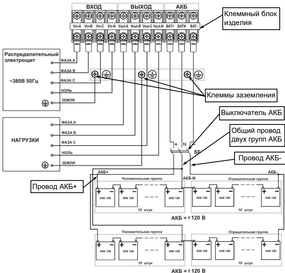
Рисунок 23.2 – Схема подключения изделия и монтажа внешних аккумуляторных батарей для SKAT-UPS 10-3/3-ON-2х(20х9), SKAT-UPS 15-3/3-ON-2х(20х9), SKAT-UPS 20-3/3-ON-2х(20х9)
