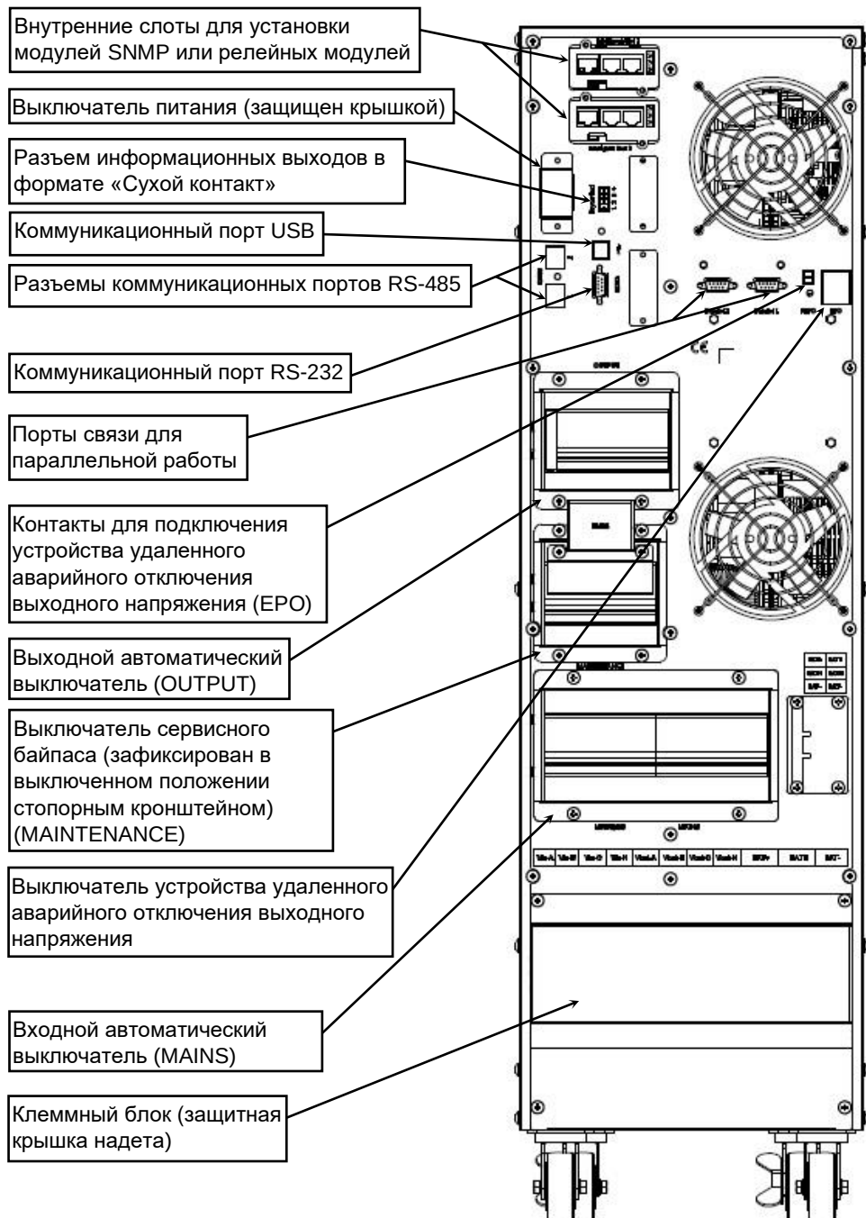
Рисунок 2.3 – Общий вид задней панели изделий SKAT-UPS 30-3/3-ON-3x(20x9) и SKAT-UPS 40-3/3-ON-2x(30x9)
