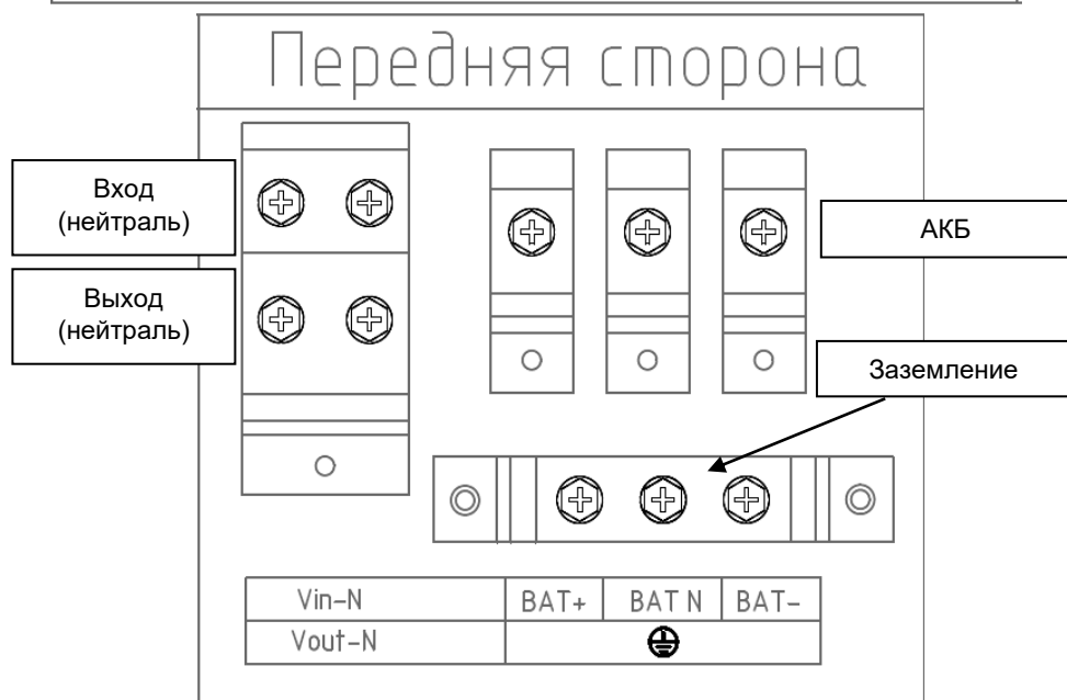
Рисунок 5 — Вид клеммных колодок изделия при трехфазном входе с питанием от одного источника, клеммы Vin и BPS соединены медными перемычками по трем фазам
