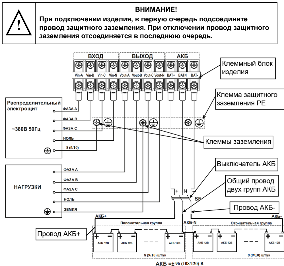
Рисунок 23 – Схема подключения изделия и монтажа аккумуляторной батареи.
