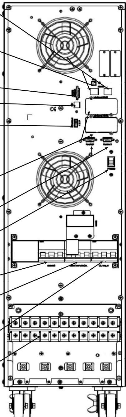
Рисунок 2.2 – Общий вид задней панели изделий SKAT-UPS 15-3/3-ON-2х(20х9) и SKAT-UPS 20-3/3-ON-2х(20х9) со снятой крышкой клеммного блока
