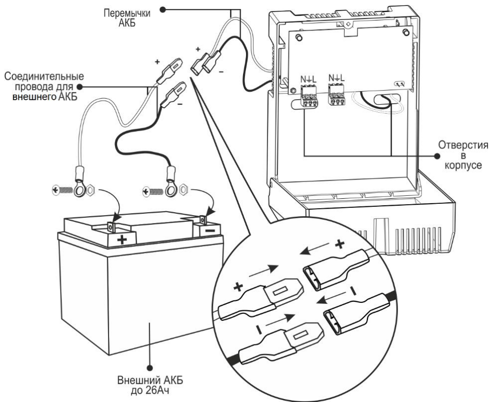
Рисунок 4 — Схема подключения внешней АКБ
