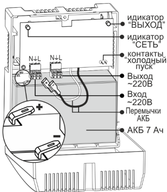
Рисунок 1 — Общий вид изделия.
