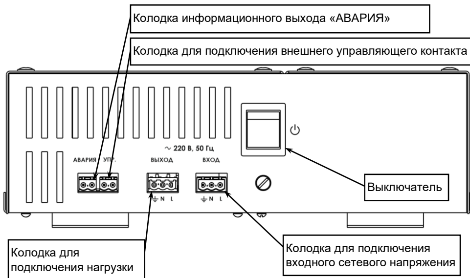
Рисунок 2 — Вид изделия со стороны подключения
