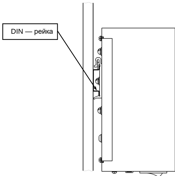
Рисунок 4 – Установка изделия на DIN-рейку
