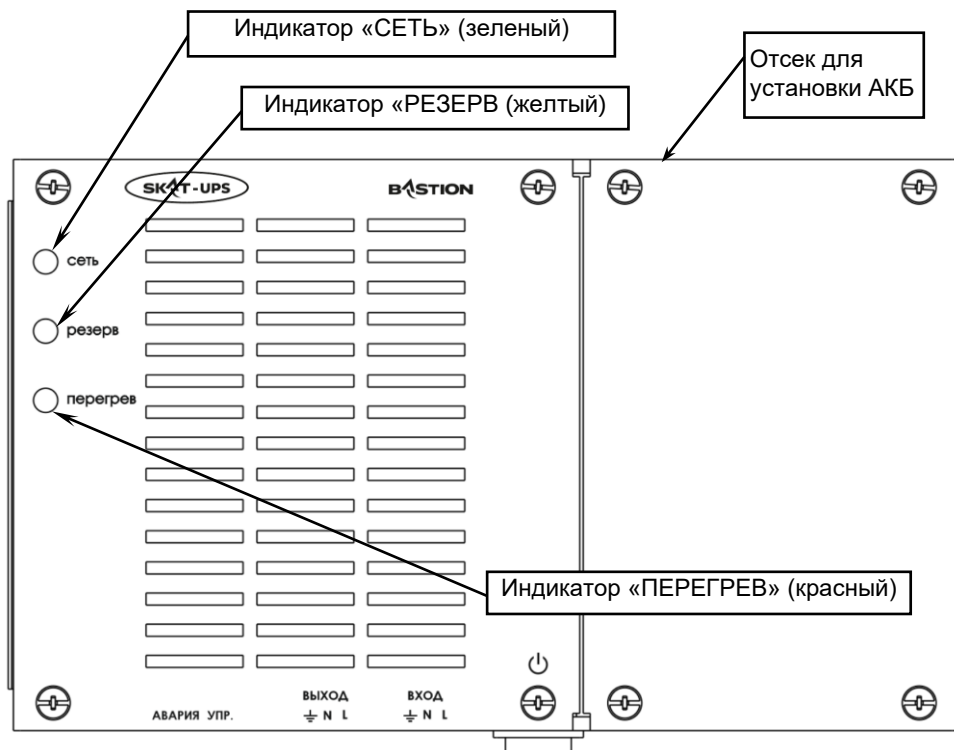
Рисунок 1 — Общий вид передней панели изделия
