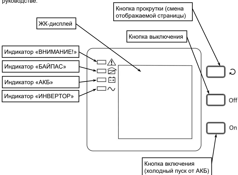
Рисунок 3 – ЖК-дисплей
