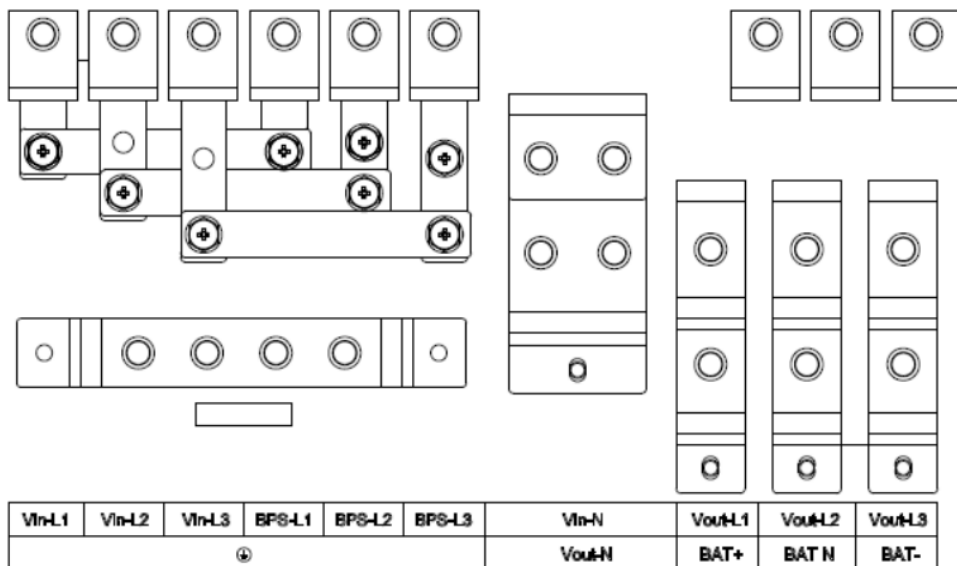
Рисунок 6 – Схема подключения изделия при одиночном входе для SKAT-UPS 100-3/3-ON, где клеммы Vin и BPS соединены медными перемычками по фазам и нейтрали
