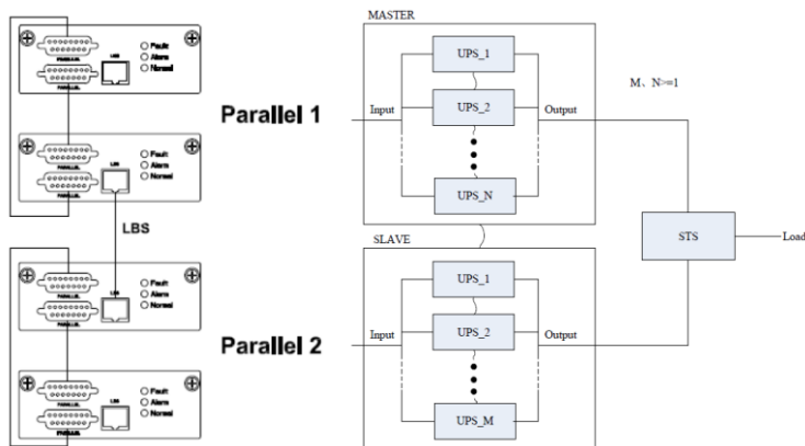
Рисунок 9 – Схема соединения изделий через LBS-кабель
