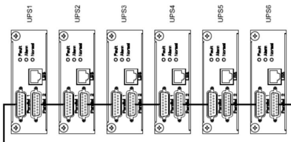
Рисунок 8 – Схема соединения изделий в «кольцо» через параллельные порты
