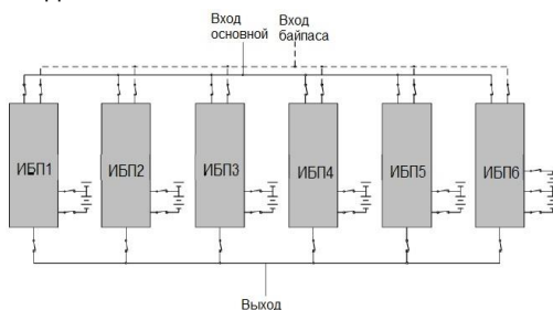
Рисунок 7 – Пример схемы подключения четырех изделий в систему параллельного резервирования с выходным распределительным шкафом.
