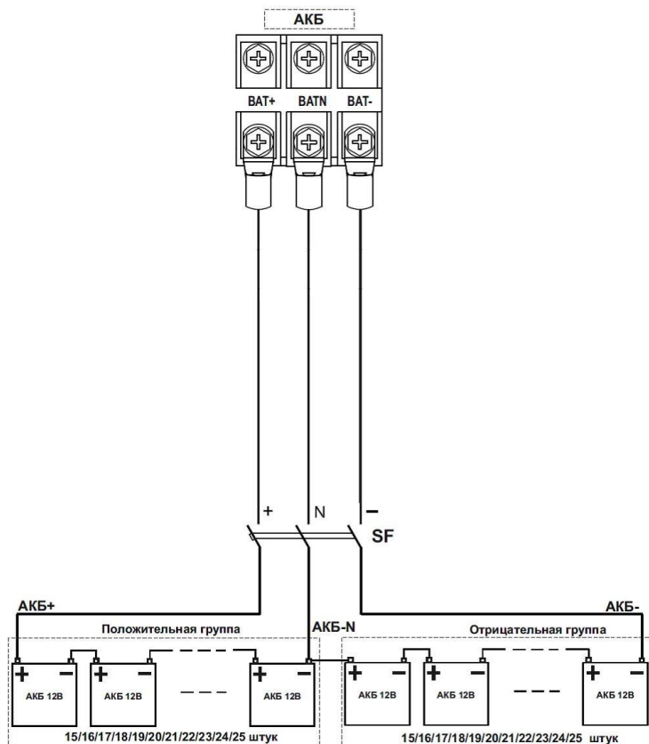
Рисунок 4 — Схема монтажа аккумуляторной батареи
