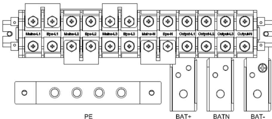
Рисунок 5 – Схема подключения изделия при одиночном входе для SKAT-UPS 80-3/3-ON, где клеммы Vin и BPS соединены медными перемычками по фазам и нейтрالي
