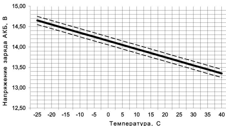
Рисунок 3 – Зависимость напряжения заряда АКБ от температуры.
