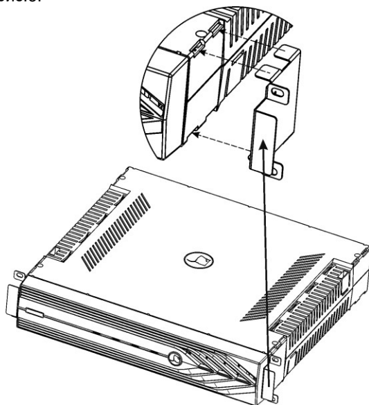
Рисунок 3 – Крепление кронштейнов для установки изделия в стойку 19"
