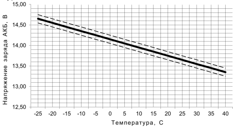
Рисунок 2 – Зависимость напряжения заряда АКБ от температуры
