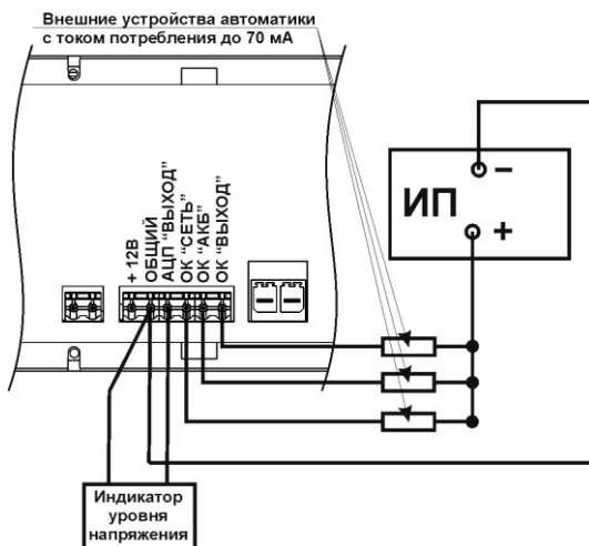
Рисунок 5 – Подключение внешних устройств автоматики
