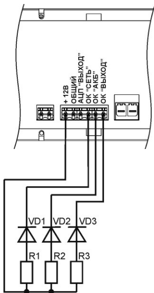
Рисунок 6 – Подключение внешних индикаторов
