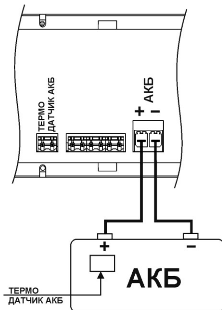
Рисунок 4 – Подключение АКБ и термодатчика АКБ.
