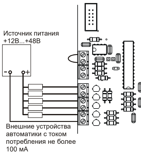
Рисунок 4.2 - Подключение внешних устройств автоматики
