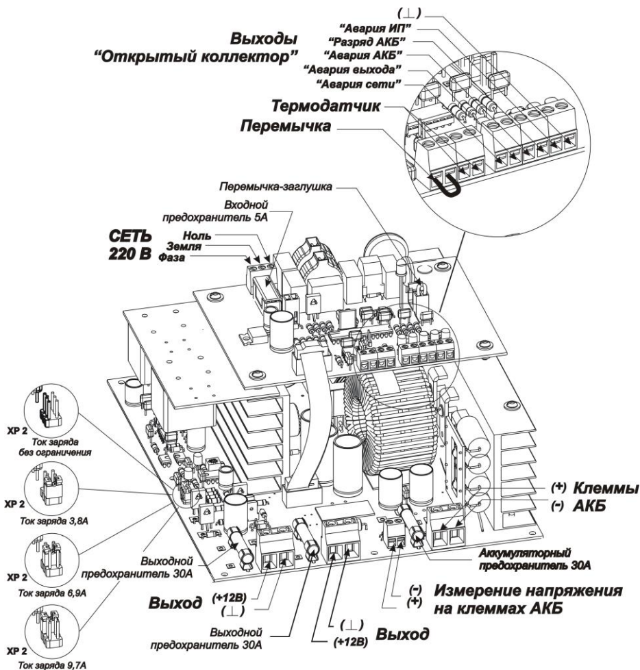
Рисунок 5 – Расположение органов коммутации, управления и защиты в зарядном устройстве
