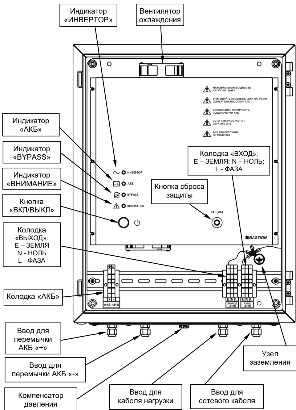
Рисунок 2 - Вид изделия с открытой дверцей.
