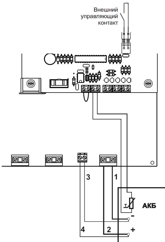
Рисунок 5 – Подключение АКБ, термодатчика и внешнего контакта
