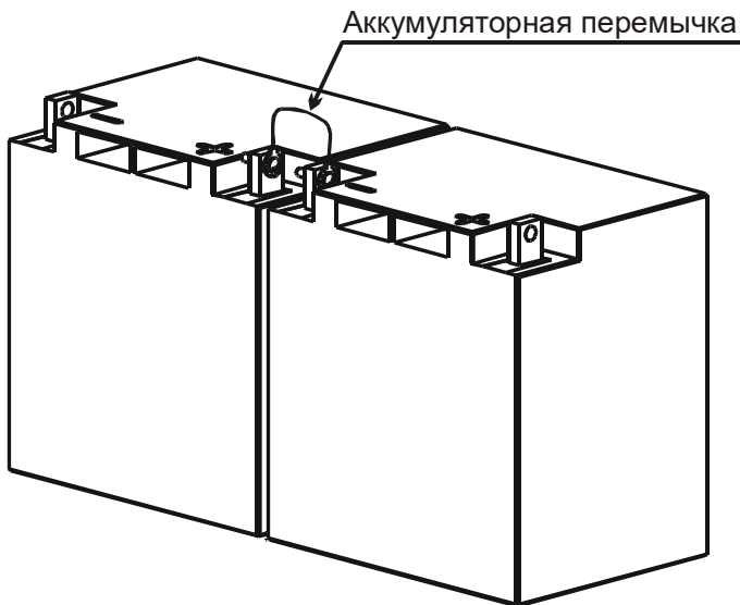
Рисунок 8 – Последовательное соединение АКБ
