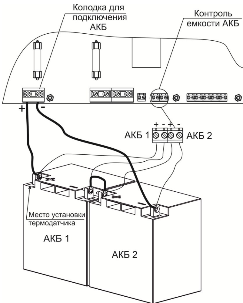
Рисунок 5 – Схема соединения аккумуляторных батарей
