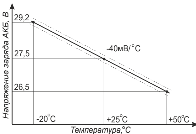
Рисунок 1 - Зависимость напряжения заряда АКБ от температуры
