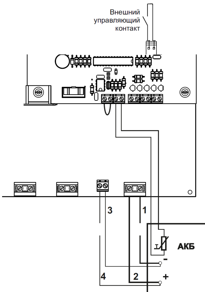
Рисунок 5 – Подключение АКБ, термодатчика и внешнего контакта
