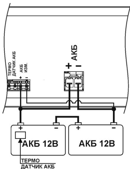
Рисунок 4 – Подключение АКБ и термодатчика АКБ.
