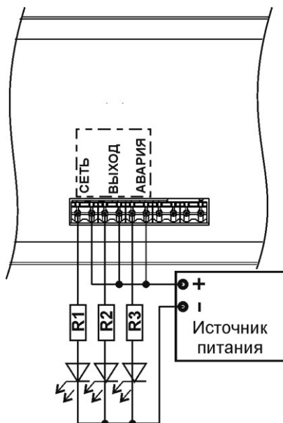
Рисунок 6 – Подключение внешних индикаторов
