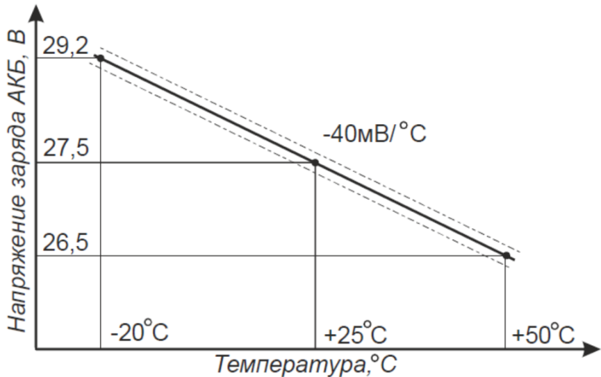
Рисунок 2 – Зависимость напряжения заряда АКБ от температуры
