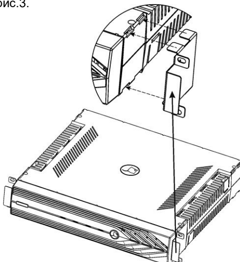
Рисунок 3 – Крепление кронштейнов для установки изделия в стойку 19"
