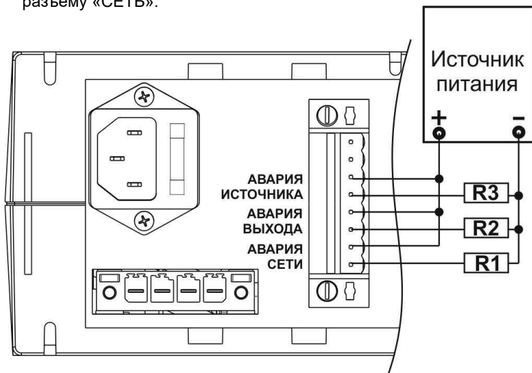
Рисунок 6 – Подключение внешних устройств автоматики
