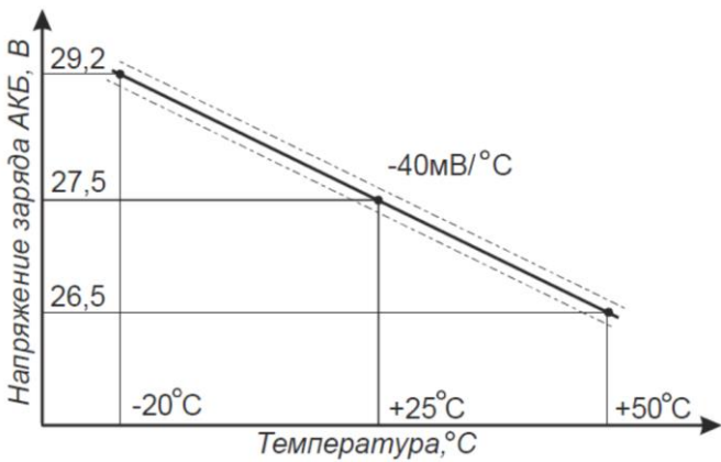
Рисунок 2 - Зависимость напряжения заряда АКБ от температуры
