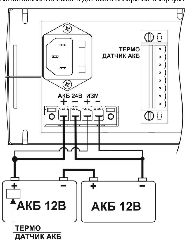
Рисунок 5 - Схема соединения аккумуляторов
