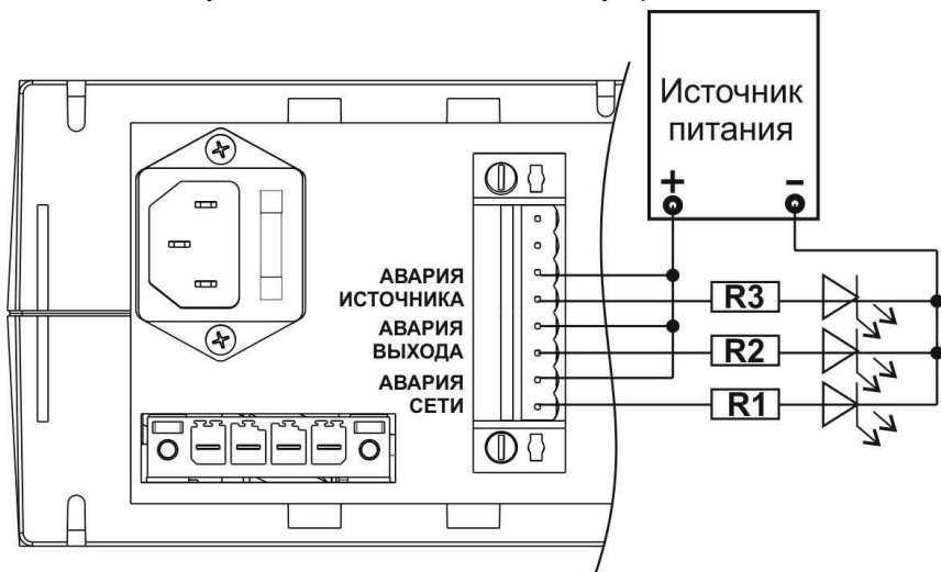
Рисунок 7 – Подключение внешних индикаторов
