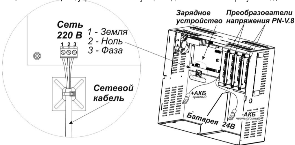
Рисунок 1 - Внешний вид изделия с открытой крышкой, подключение сетевых проводов и провода заземления
