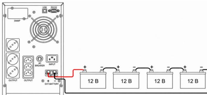
Рисунок 3 – Пример подключения цепи АКБ к ИБП модели SNR-UPS-LID-2000-SPS.
