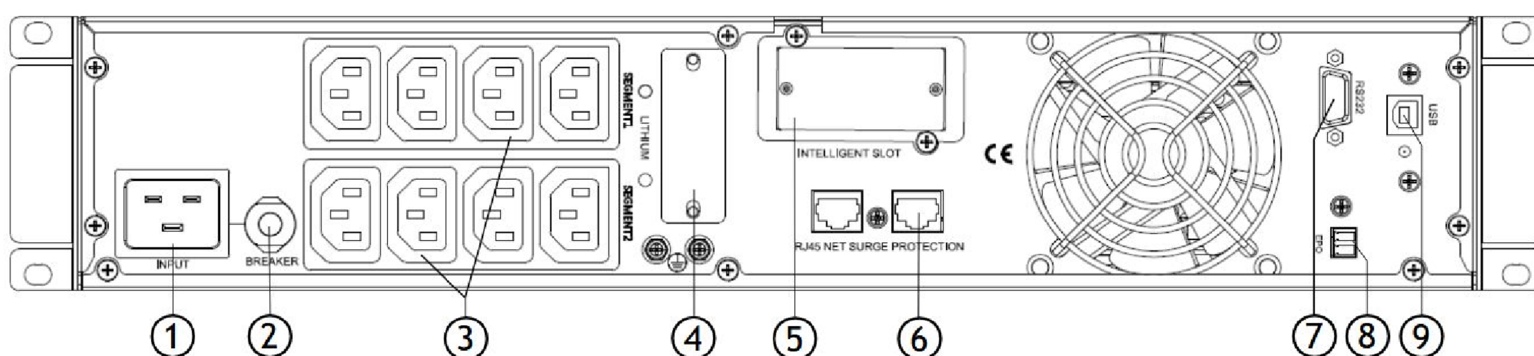
Рис.3 — Общий вид моделей мощностью 2000 ВА
