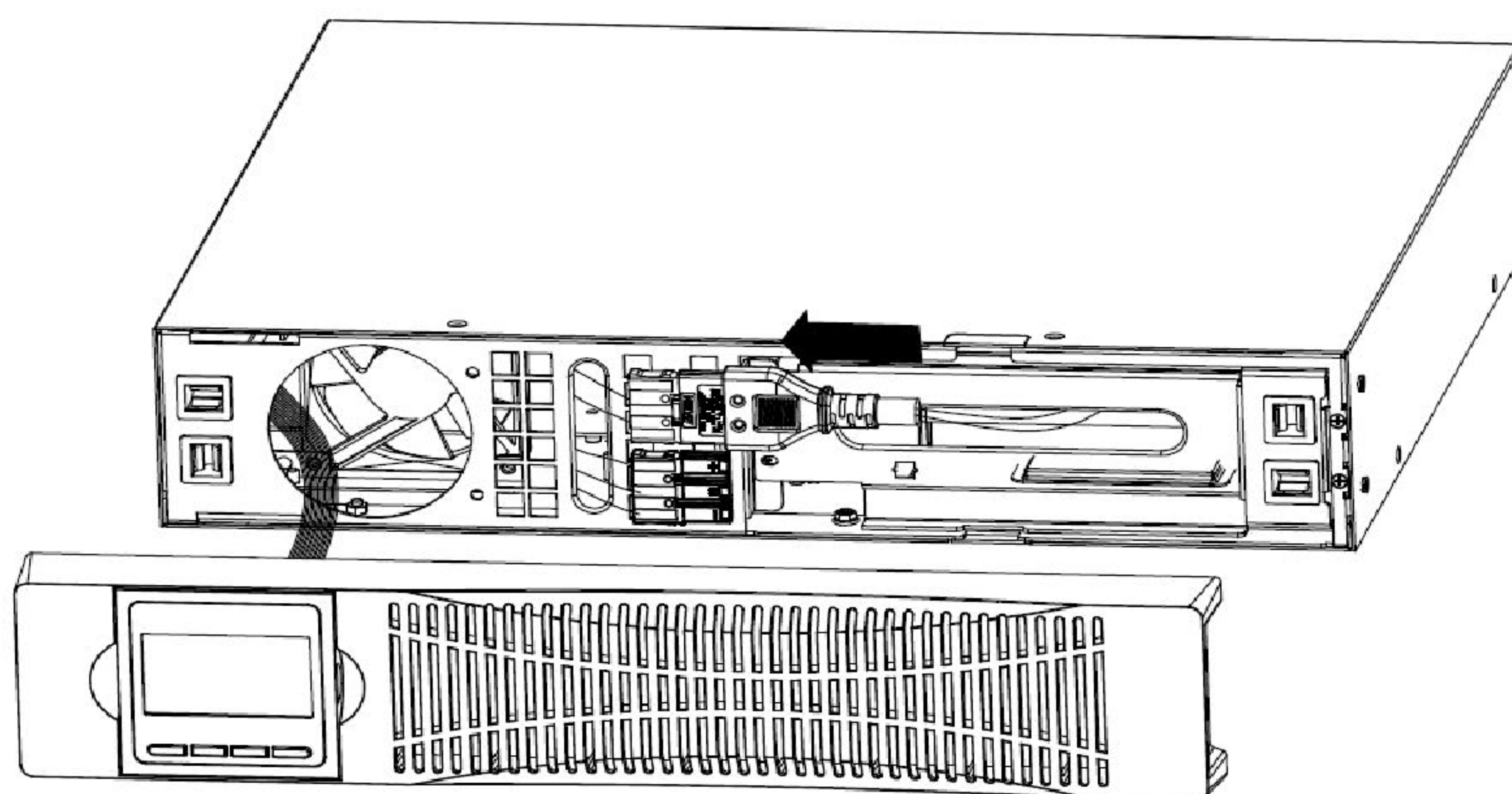
Рис. 12 — Подключение разъема встроенных аккумуляторов
