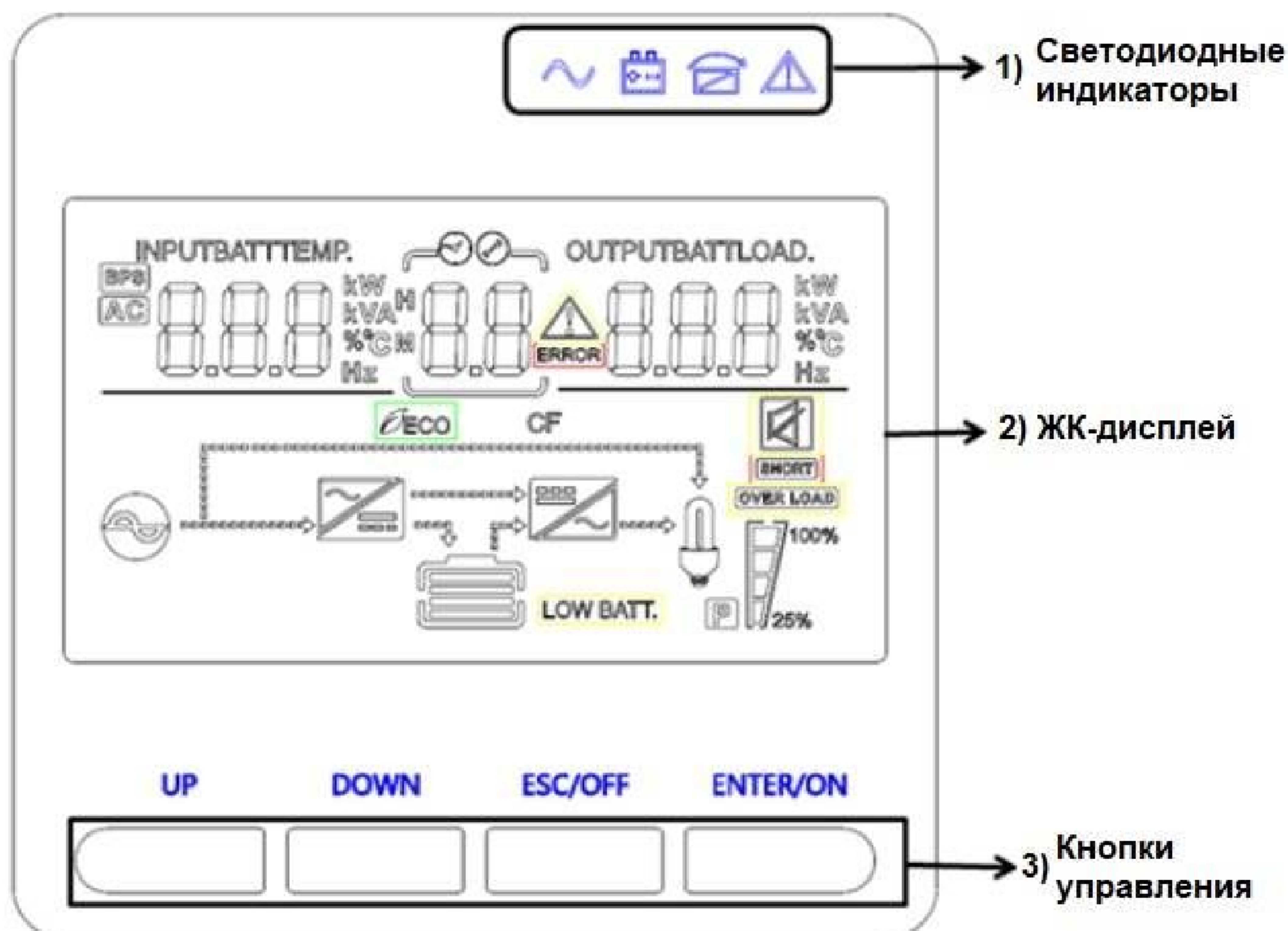
Рис. 13 — Общий вид панели управления
