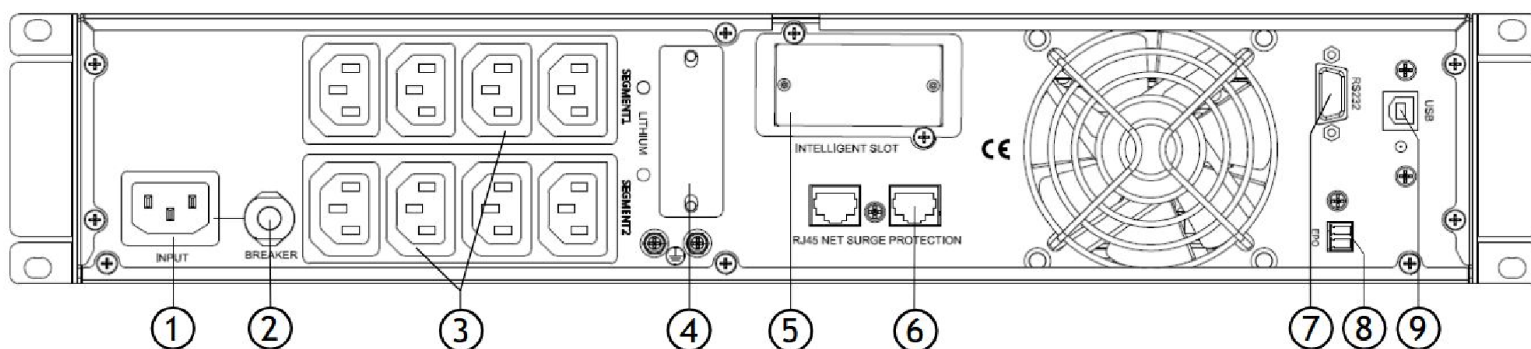
Рис.2 — Общий вид моделей мощностью 1000 ВА
