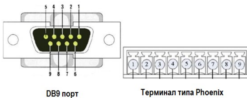
Рисунок 6.2 Сухие контакты
