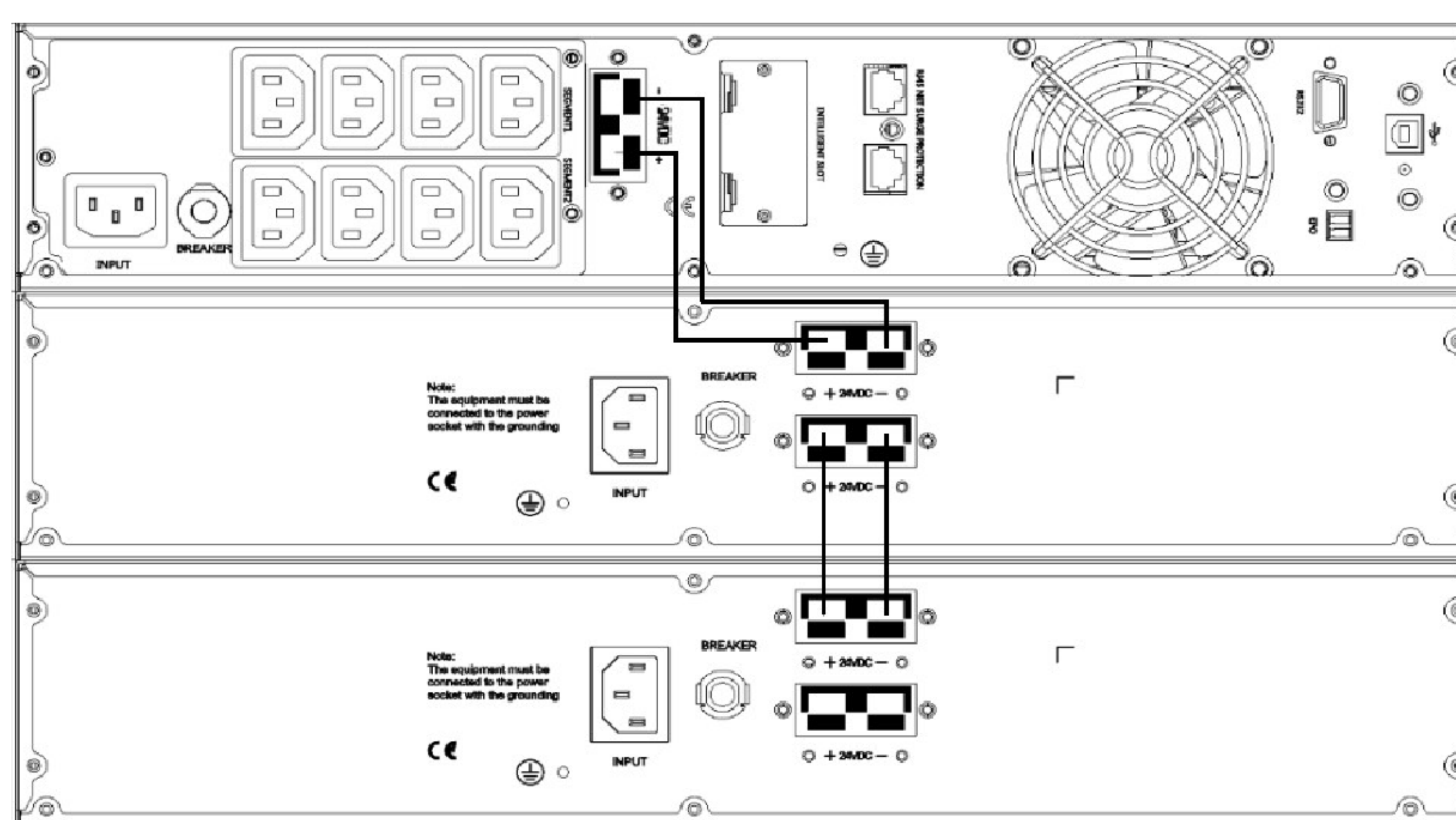
Рис.14 — Схема подключения дополнительных блоков батарей
