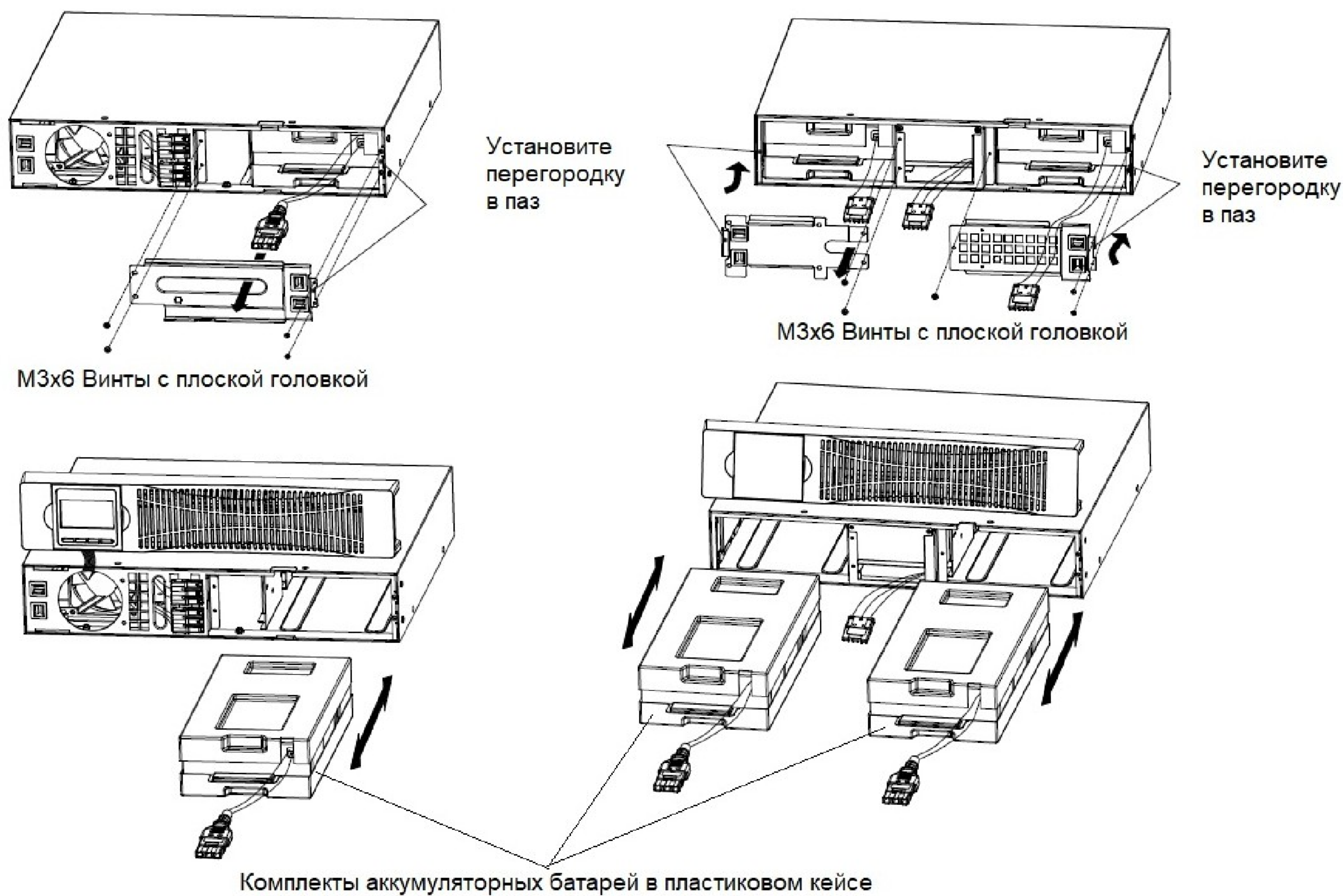
Рис.21 — Замена аккумуляторных батарей в ИБП и дополнительном блоке батарей
