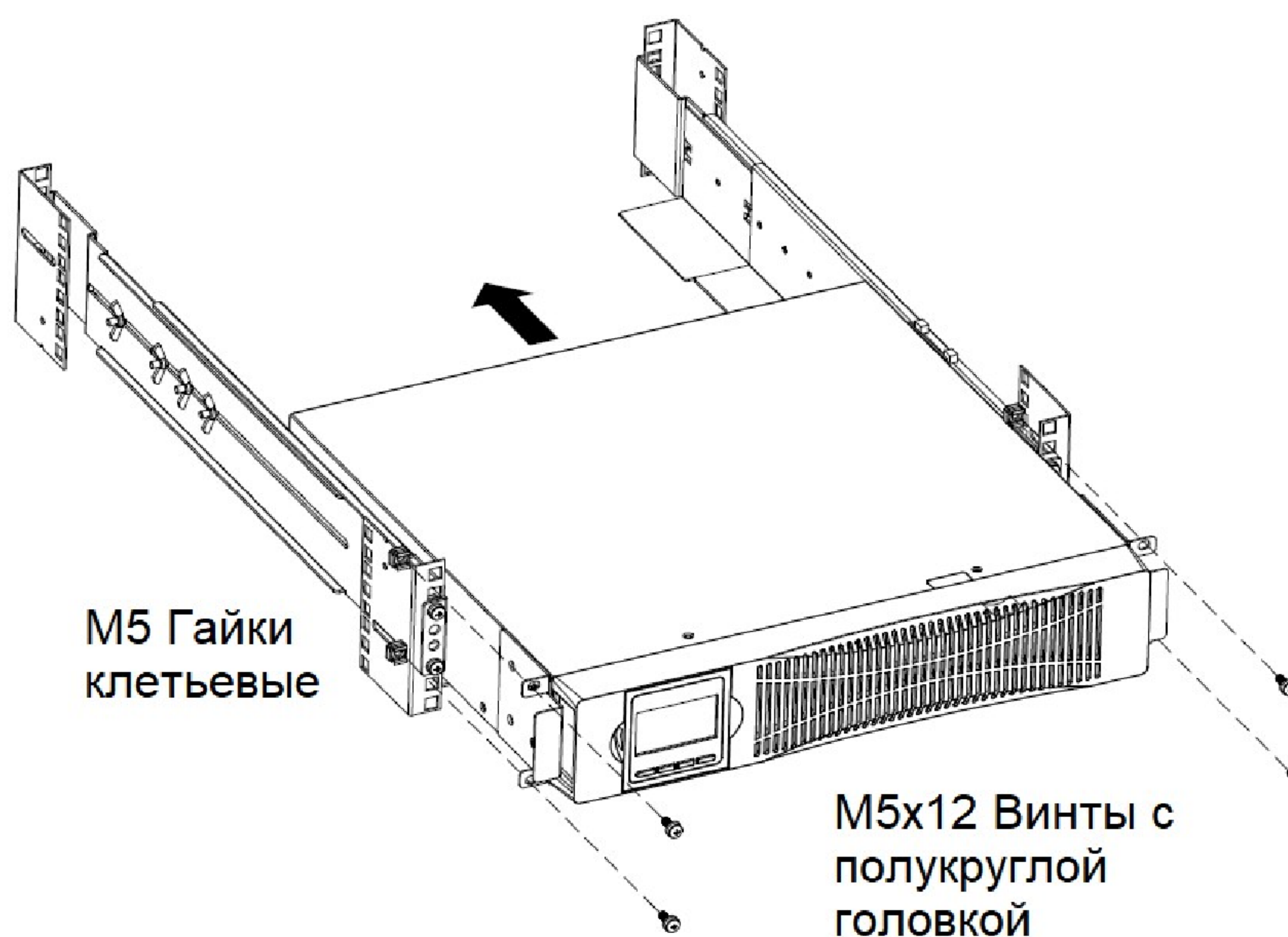
Рис.8 — Установка ИБП в стойку 19"
