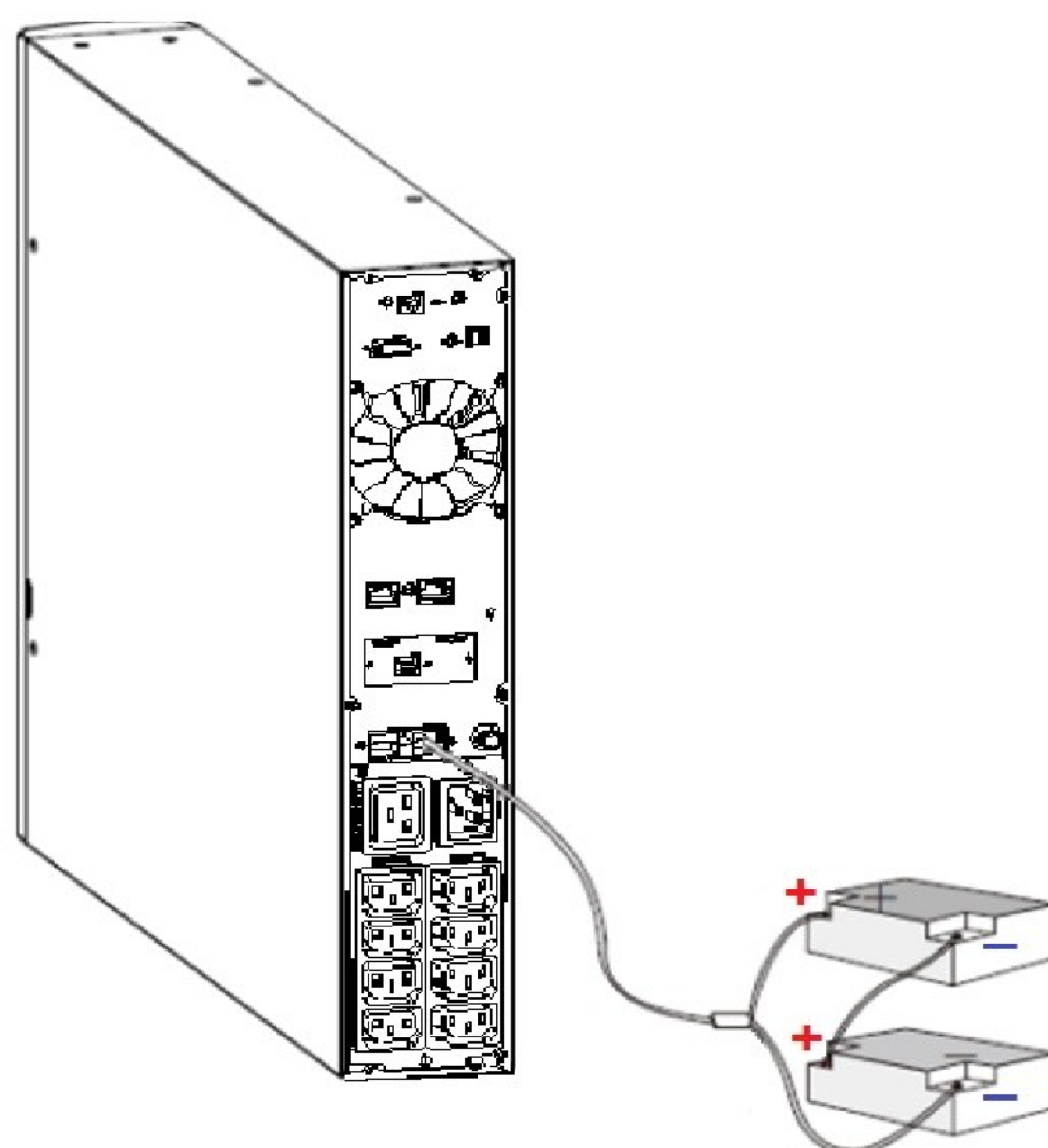
Рис.15 — Схема подключения внешних аккумуляторных батарей (-X, -XL)
