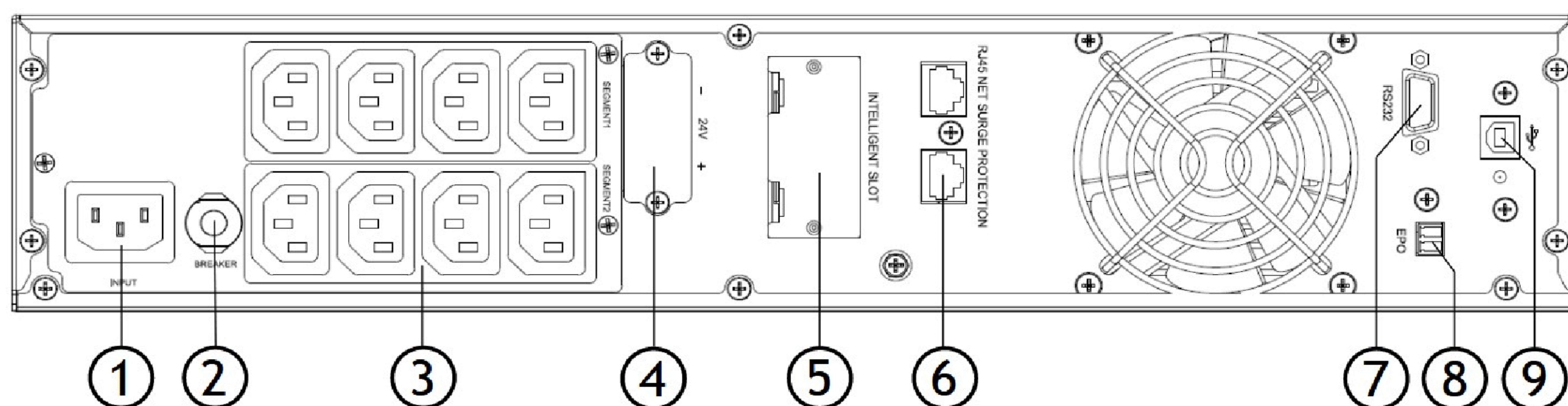
Рис.2 — Общий вид моделей мощностью -1000 ВА и -1500 ВА
