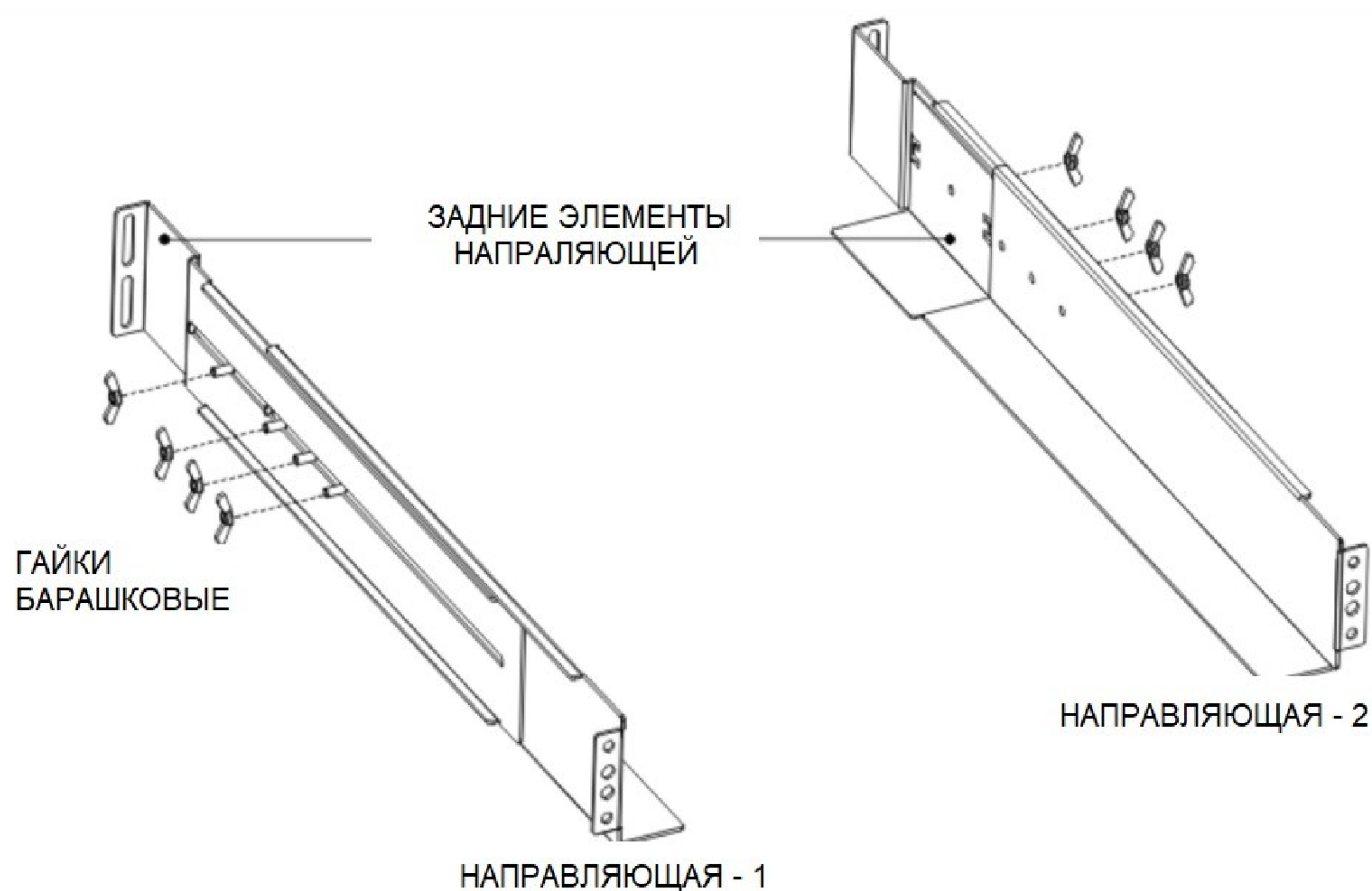
Рис.5 — Сборка направляющих
