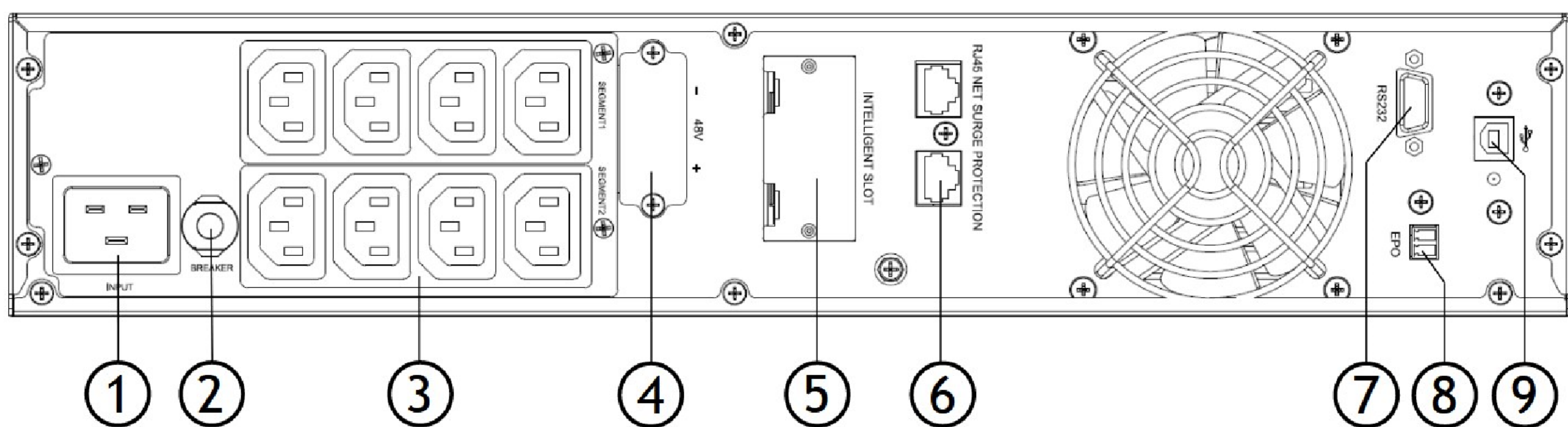
Рис.3 — Общий вид моделей мощностью -2000 ВА
