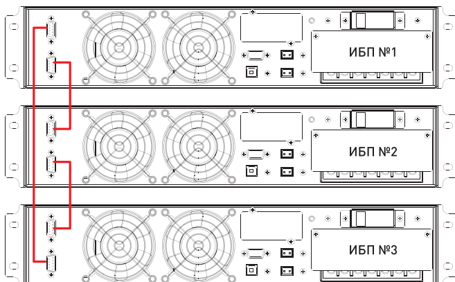
Рис. 16 - Подключение коммуникационных кабелей 3х ИБП
