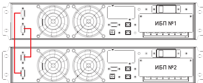
Рис. 15 - Подключение коммуникационных кабелей 2х ИБП
