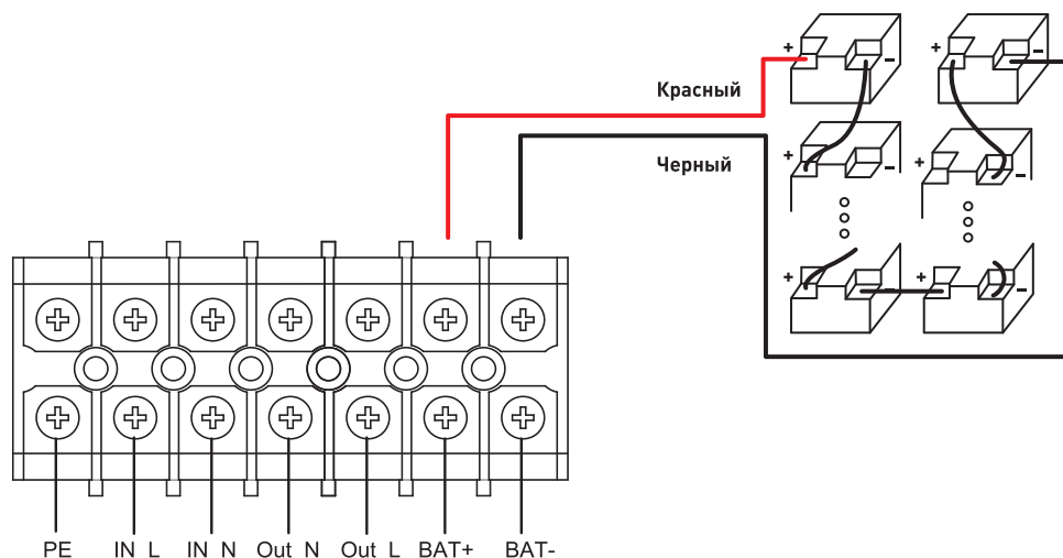
Рис. 5 - Схема подключения внешних аккумуляторных батарей к ИБП
