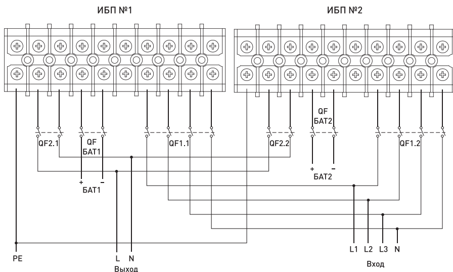
Рис. 14 - Схема параллельного подключения ИБП 3:1
