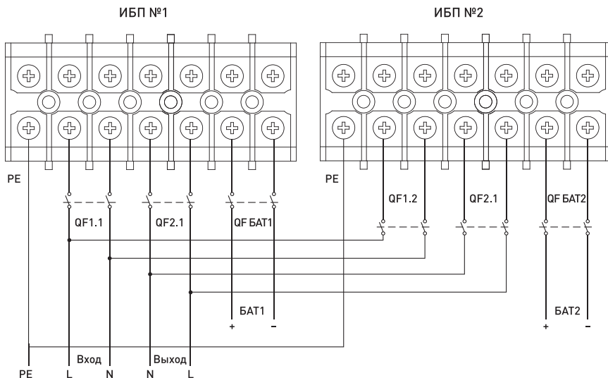
Рис. 13 - Схема параллельного подключения ИБП 1:1
