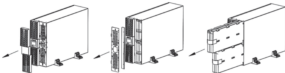
Рис. 31 - Последовательность действий при замене АКБ в ИБП серий SW900G4-RTB
