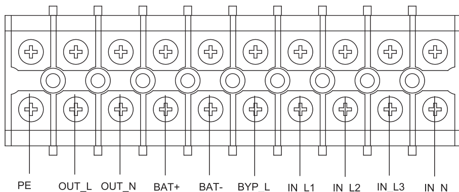
Рис. 4 - Клеммная колодка ИБП 10кВА вариант подключения 3:1
