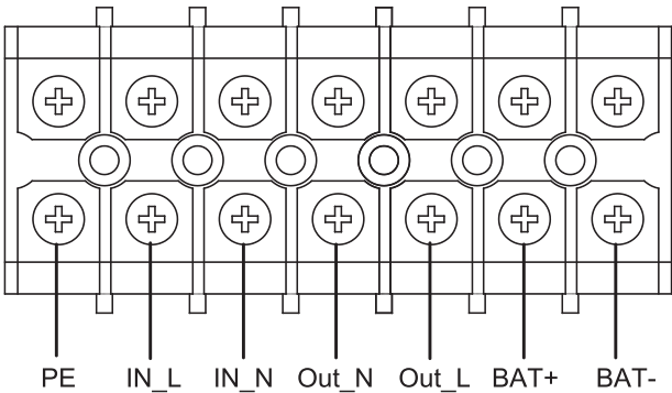
Рис. 3 - Клеммная колодка ИБП вариант подключения 1:1
