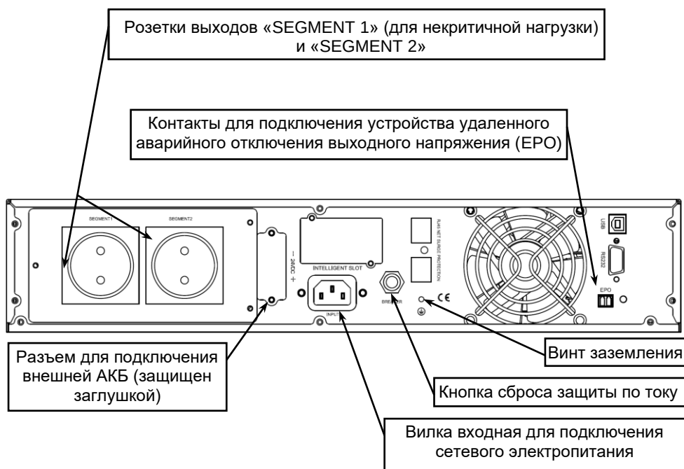
Рисунок 2 – Общий вид задней панели изделия
