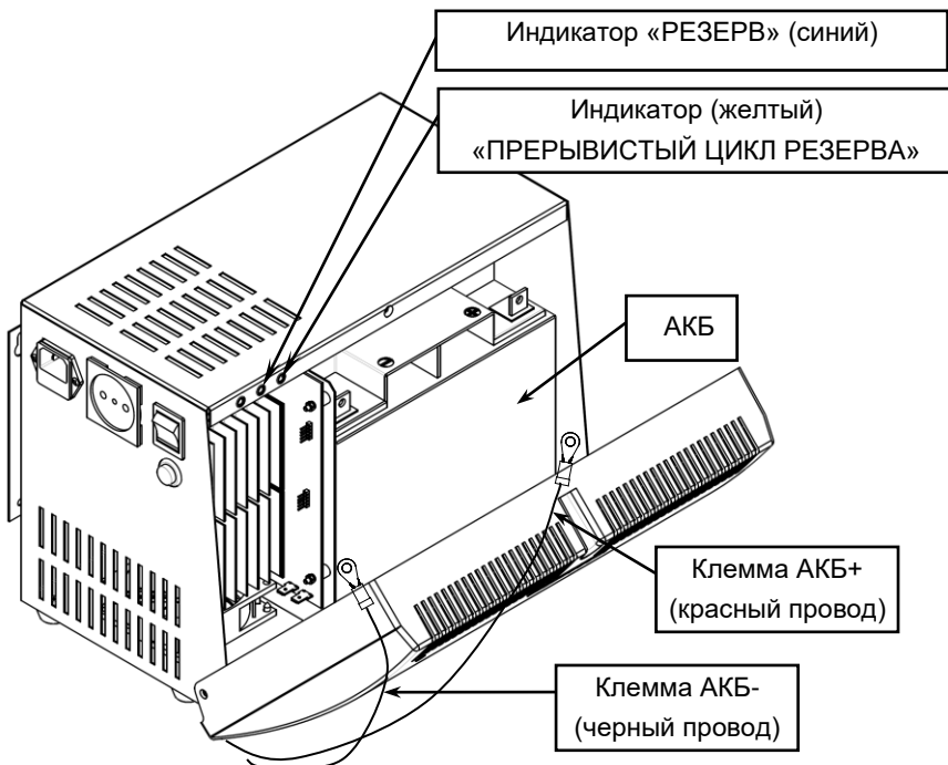
Рисунок 3 – Общий вид изделия с приоткрытой крышкой и установленной АКБ
