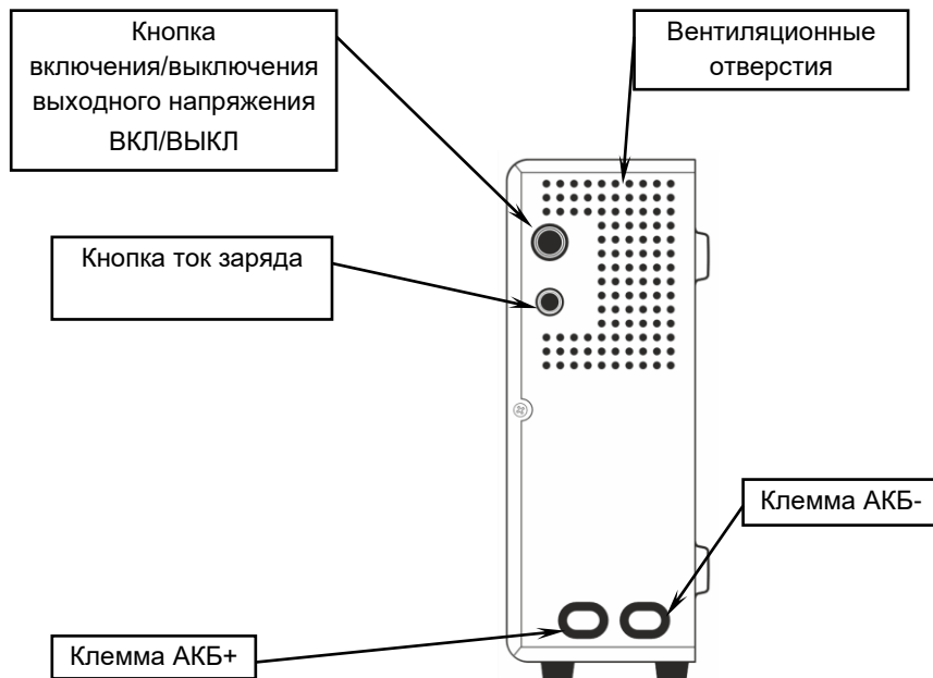
Рисунок 2 – Вид изделия слева
